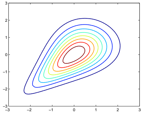
(d) Clayton copula: \theta = 1
