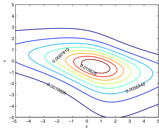
(d) Contour Plot: GTL-nJoe
