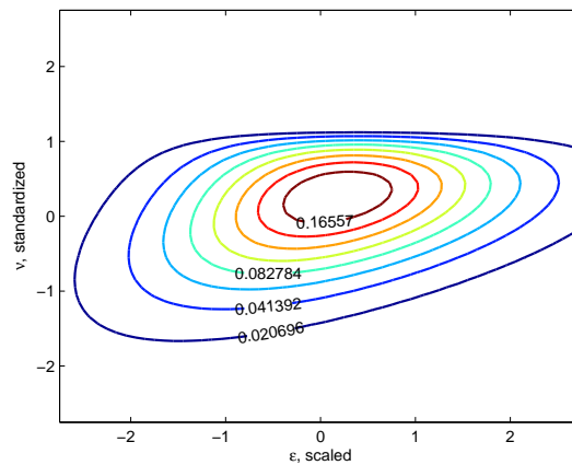
(d) Contour plot: GTL-Clayton
