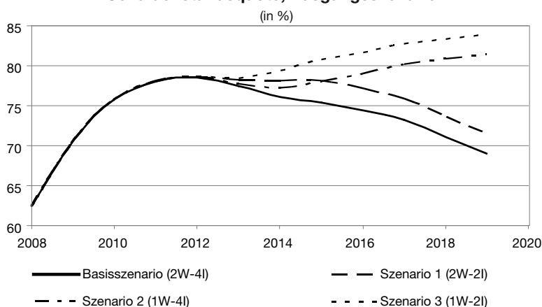
Abbildung 1 Schuldenstandsquote, Ausgangsszenarien
