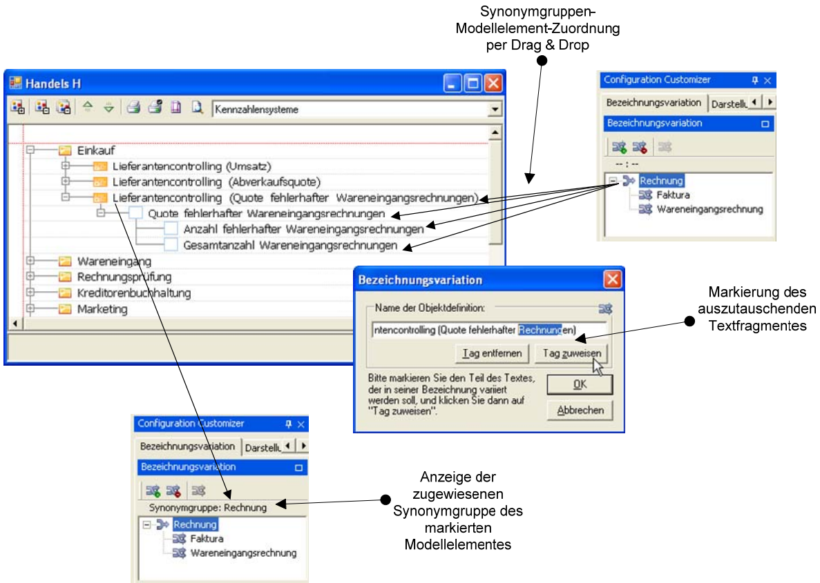
Abb. 52: Zuweisung von Synonymgruppen zu Modellelemente
