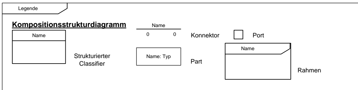
Abb. 3.28: Legende zu den Elementen des Kompositionsstrukturdiagrammes
