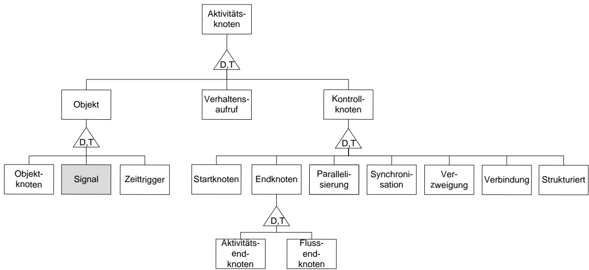
Abb. 3.20 Aktivitätsknoten im Metamodell des Aktivitätsdiagrammes
