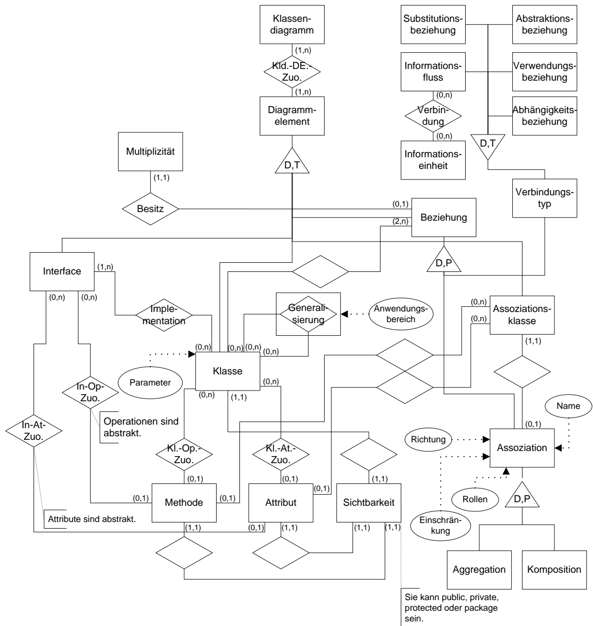
Abb. 3.22: Metamodellausschnitt des Klassendiagrammes
