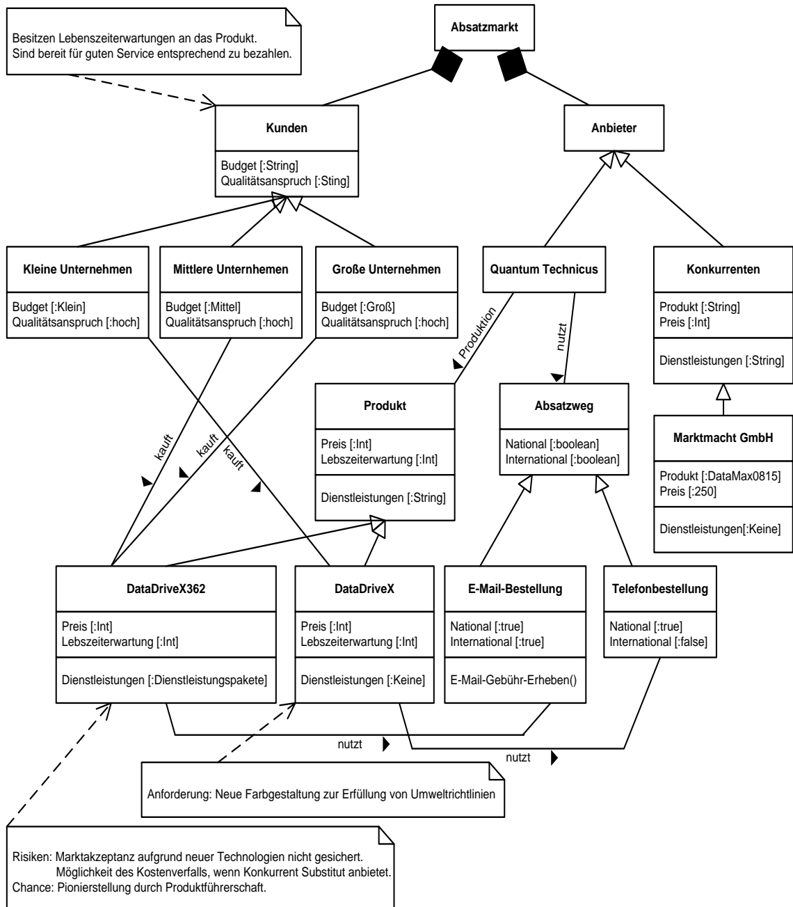
Abb. 4.24: Beschreibung des Absatzmarktes
