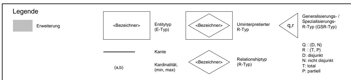
Abb. 3.11: Metamodell Anforderungenmodell
