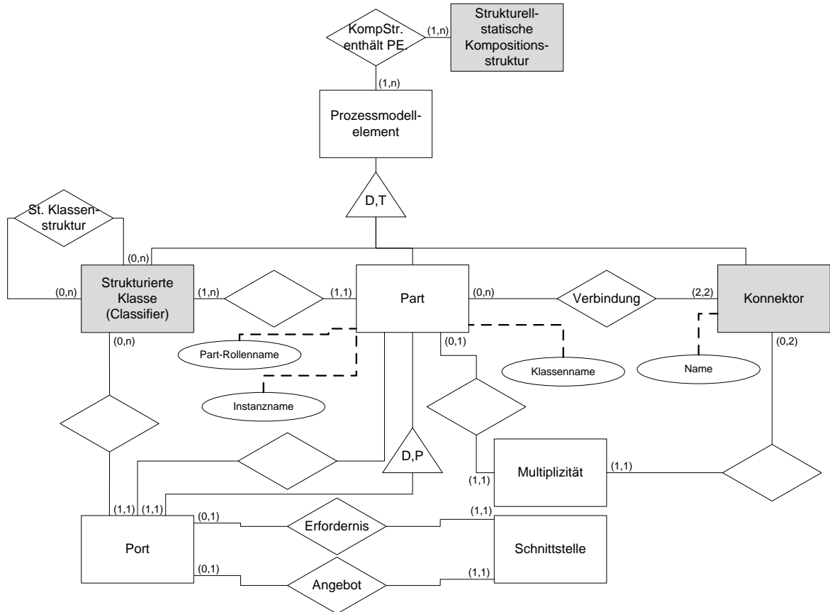
Abb. 3.27: Metamodelausschnitt der strukturell-statischen Kompositionsstrukturen
