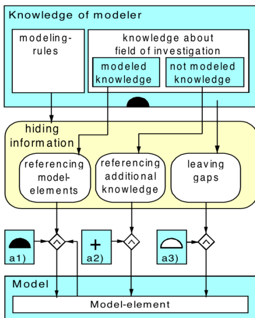
Abb. 3.85: Kennzeichnung von Vagheit in SeeMe
