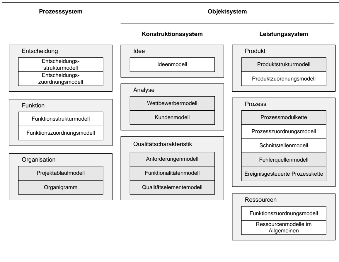
Abb. 3.7: Modellierungstechniken des Service Systems Engineering
