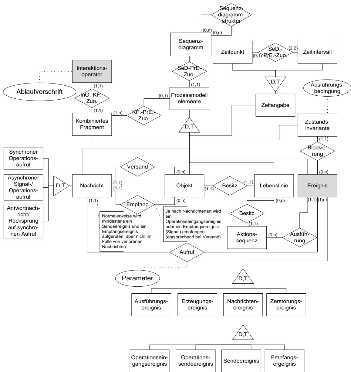
Abb. 3.23: Metamodellausschnitt des Sequenzdiagrammes
