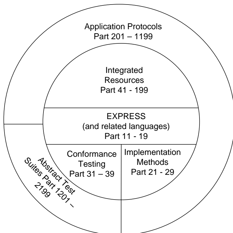
Abb. 2.7: STEP Dokumentenarchitektur
