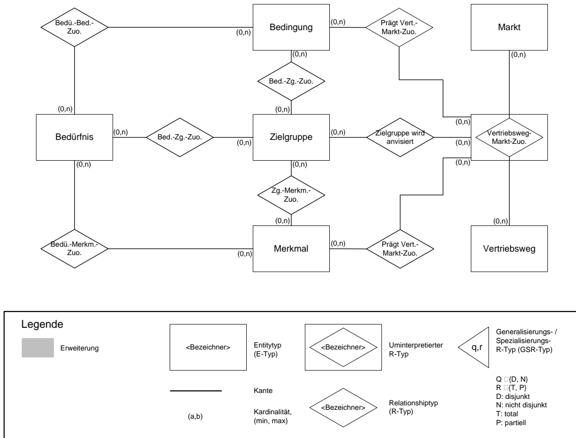
Abb. 3.10: Metamodell Kundenmodell
