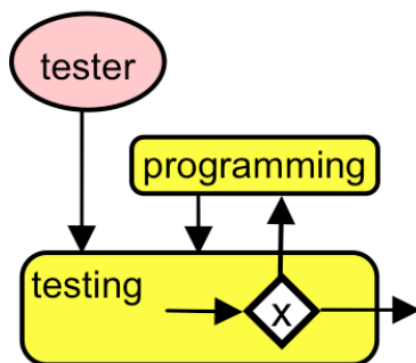
Abb. 3.78: Eingesetzter SeeMe-Konnektor
