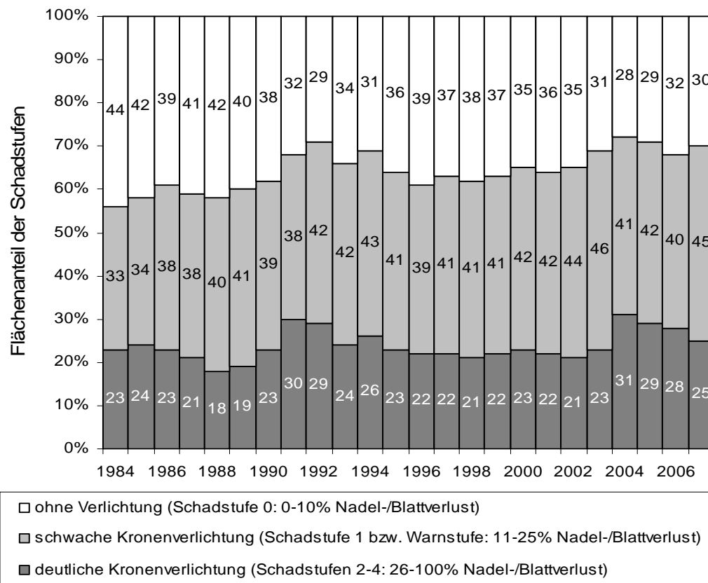
Abbildung 2: Die Ergebnisse der Waldzustandsinventuren 1984 bis 2007 in der BRD für alle Baumarten (bis 1989 ohne neue Länder) 171
