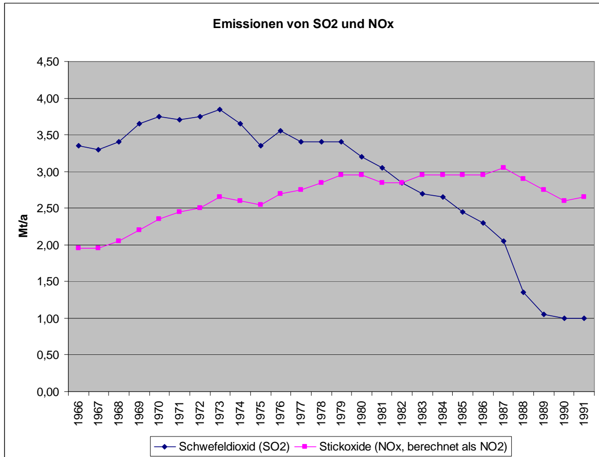
Abbildung 3: Emissionen von SO 2 und NO x in der Bundesrepublik (nur alte Länder) 198
