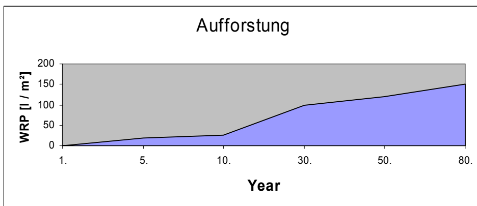
Abbildung 7 Wasserrückhaltevolumen einer natürlichen Maßnahme
