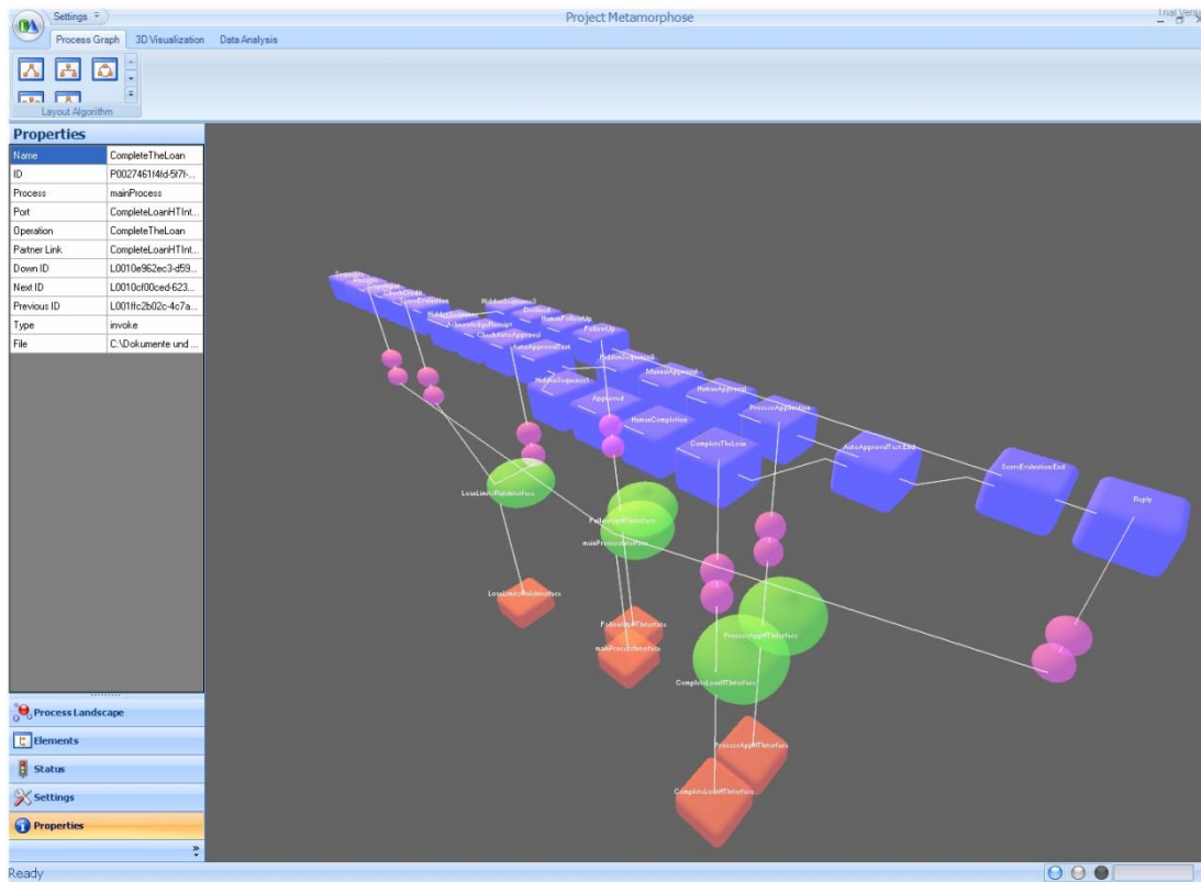
Abbildung 10: Prototypische Implementierung
