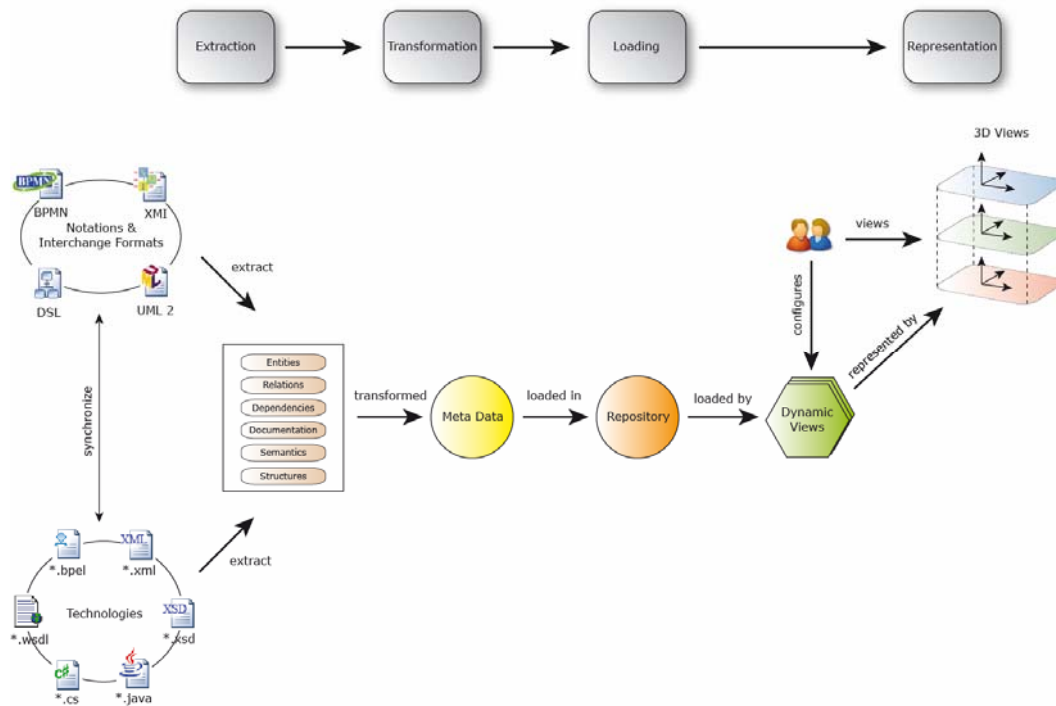
Abbildung 9: Die ETLR-Visualisierungspipeline
