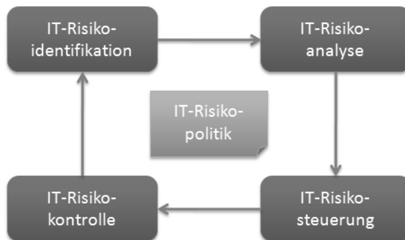
Abbildung 16: IT-Risikomanagementprozess
