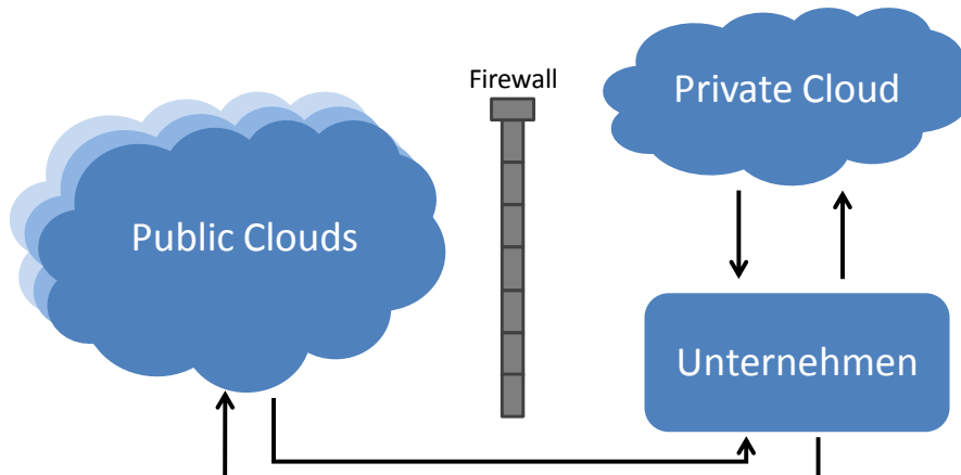
Abbildung 4: Hybrid Cloud
