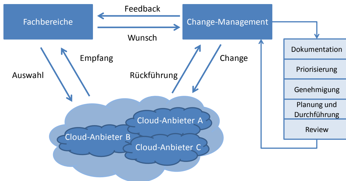
Abbildung 12: Change-Management-Prozess
