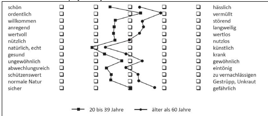
Abb. 4.3.8.1: Polaritätsprofil Brachflächen
