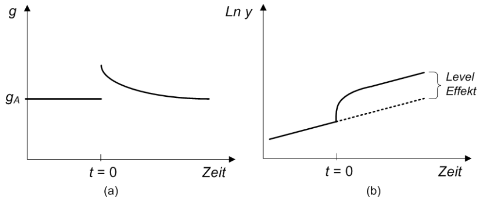
Abbildung 2 – (a) Auswirkung einer Erhöhung des Ideenbestands zu t=0 auf g_A (b) Auswirkung einer Erhöhung des Ideenbestands zu t=0 auf y Quelle: Eigene Darstellung in Anlehnung an Jones (2002, S.108) (a) und Jones (2002, S.43) (b)
