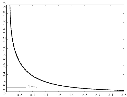
5.1: BAC
