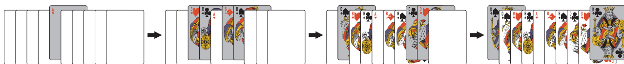
Abb. 15: Anordnungsfolge für die maximale Vermischung eines Beispiels mit 10 Karten und vier Fraktionen unterschiedlicher Größe
