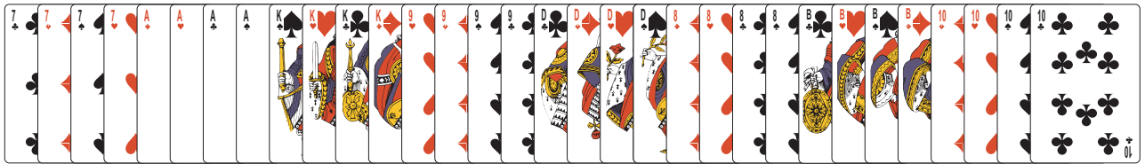
Abb. 9: Unvermischtheit aller Fraktionen 20
