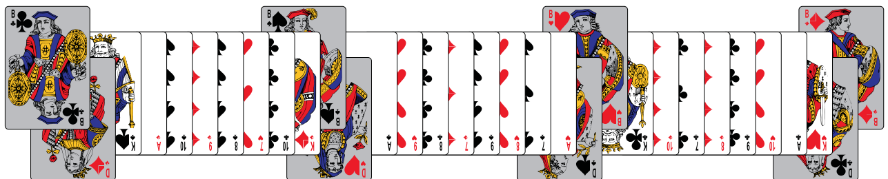
Abb. 10: Maximalabstände verschiedener Fraktionen
