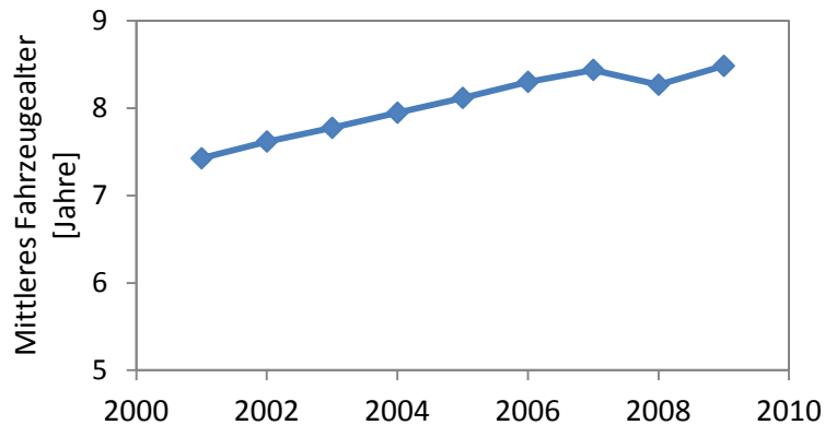
Abbildung 18: Entwicklung des mittleren Fahrzeugalters 2001 – 2009
