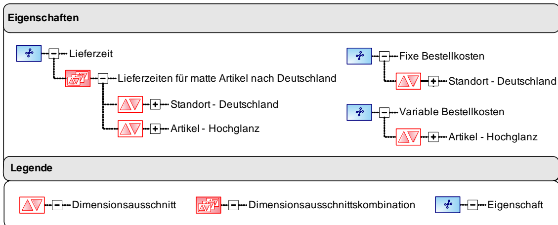
Abbildung 22: Zuweisung von Serviceräumen zu Eigenschaften
