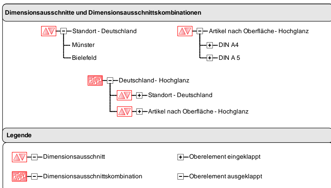
Abbildung 21: Definition der Dimensionsausschnitte und Dimensionsausschnittskombinationen
