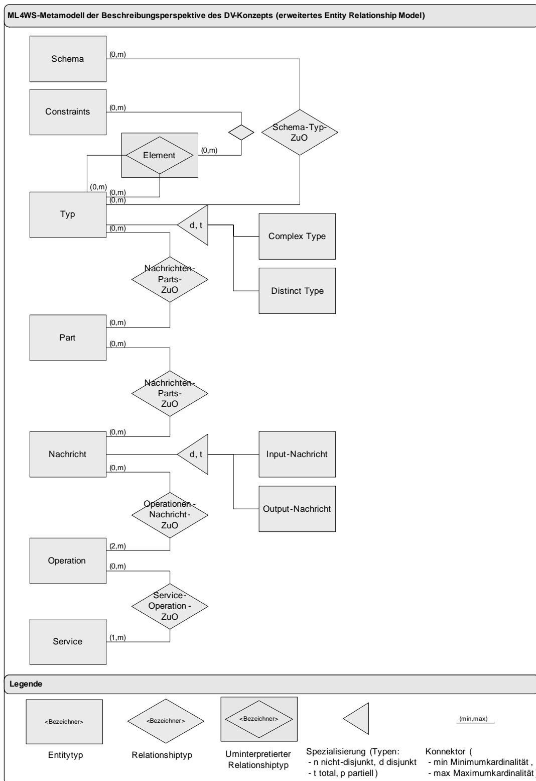
Abbildung 14: ML4WS-Metamodell der Beschreibungsperspektive des DV-Konzepts
