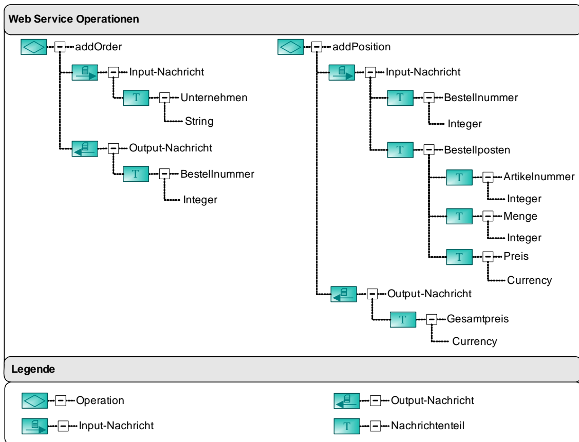
Abbildung 29: Aufgliedern der Operationen in Nachrichten
