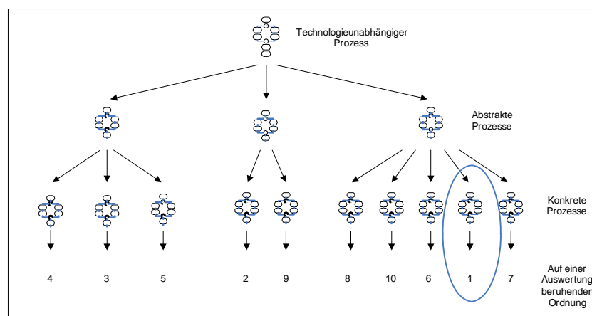
Abbildung 13: Bestimmung der einzubindenden Web Services anhand eines technologieunabhängigen Prozesses
