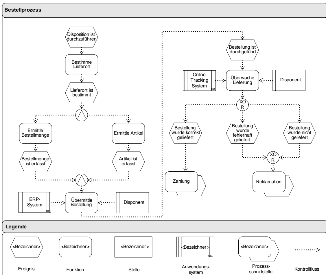
Abbildung 18: Prozessmodell zum Bestellprozess
