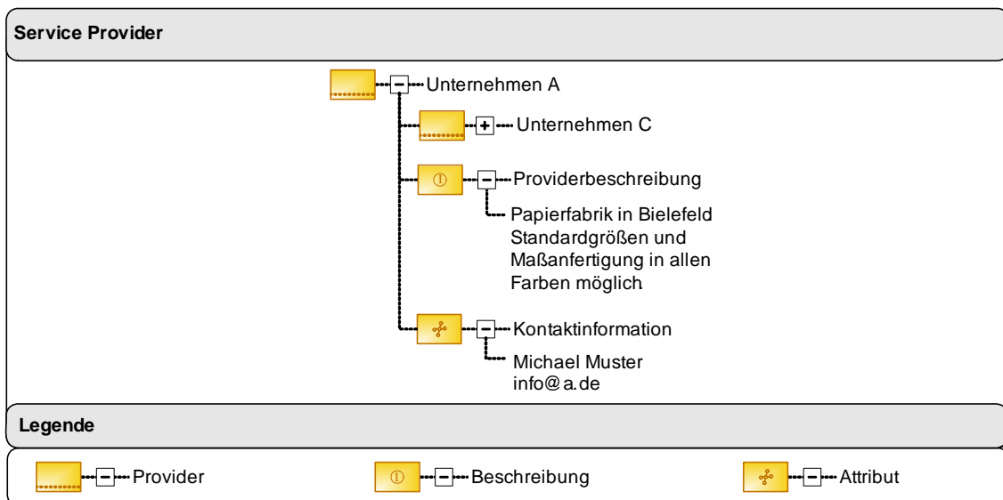
Abbildung 30: Erweiterung des Service Providers im DV-Konzept
