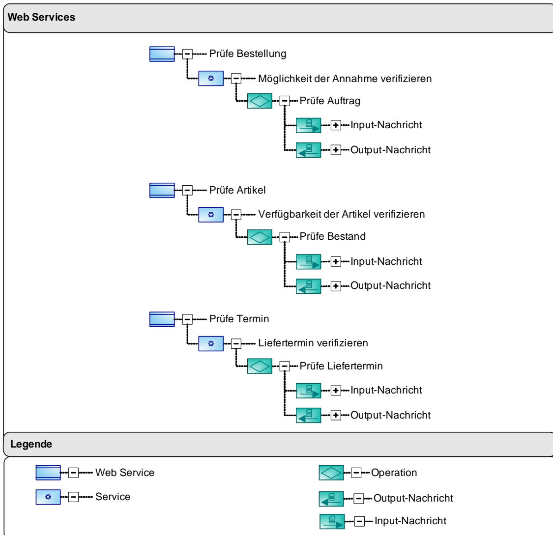
Abbildung 32: Auszug aus der Web Service-Spezifikation
