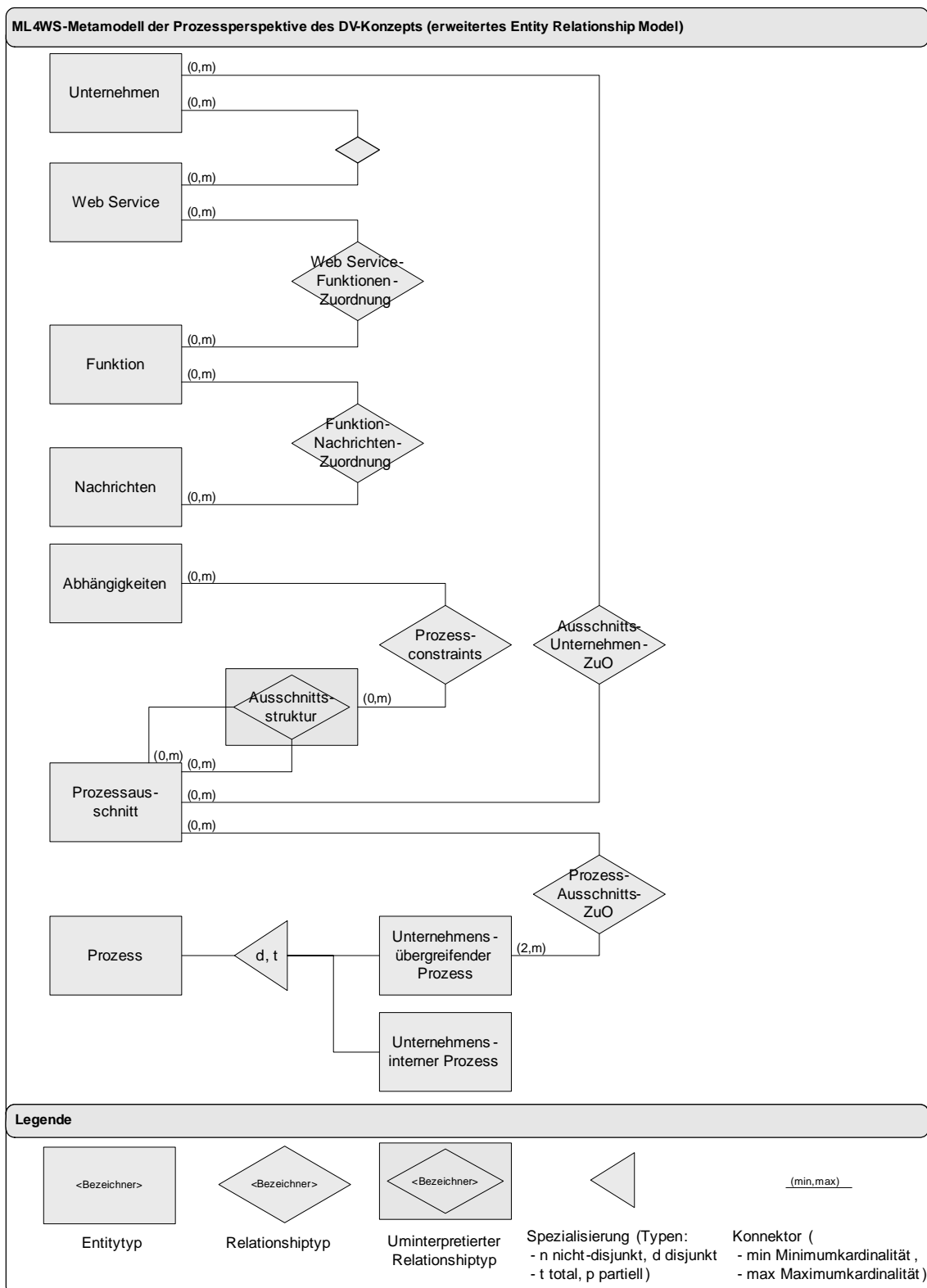
Abbildung 16: ML4WS-Metamodell der Prozessperspektive des DV-Konzepts
