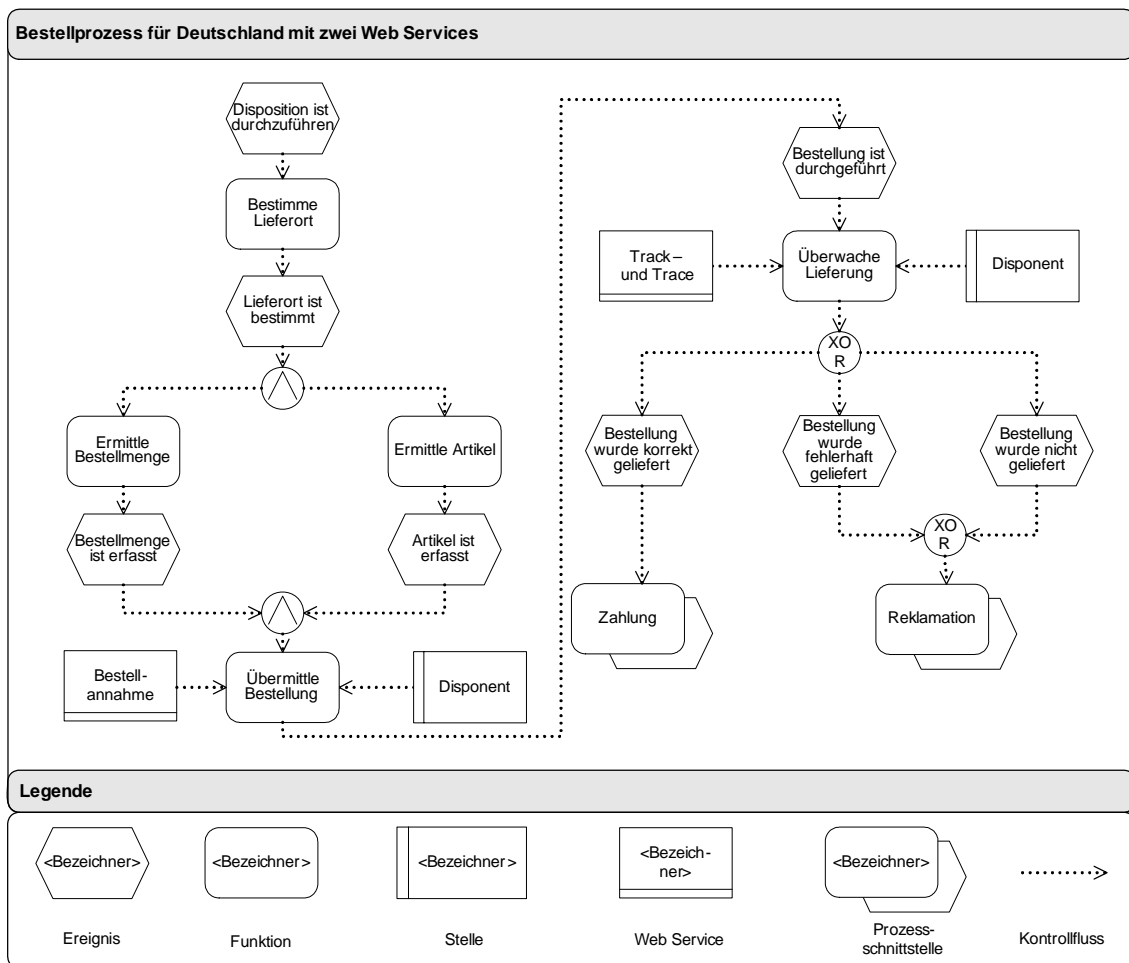
Abbildung 25: Umsetzung des unabhängigen Bestellprozesses in einen abstrakten Prozess
