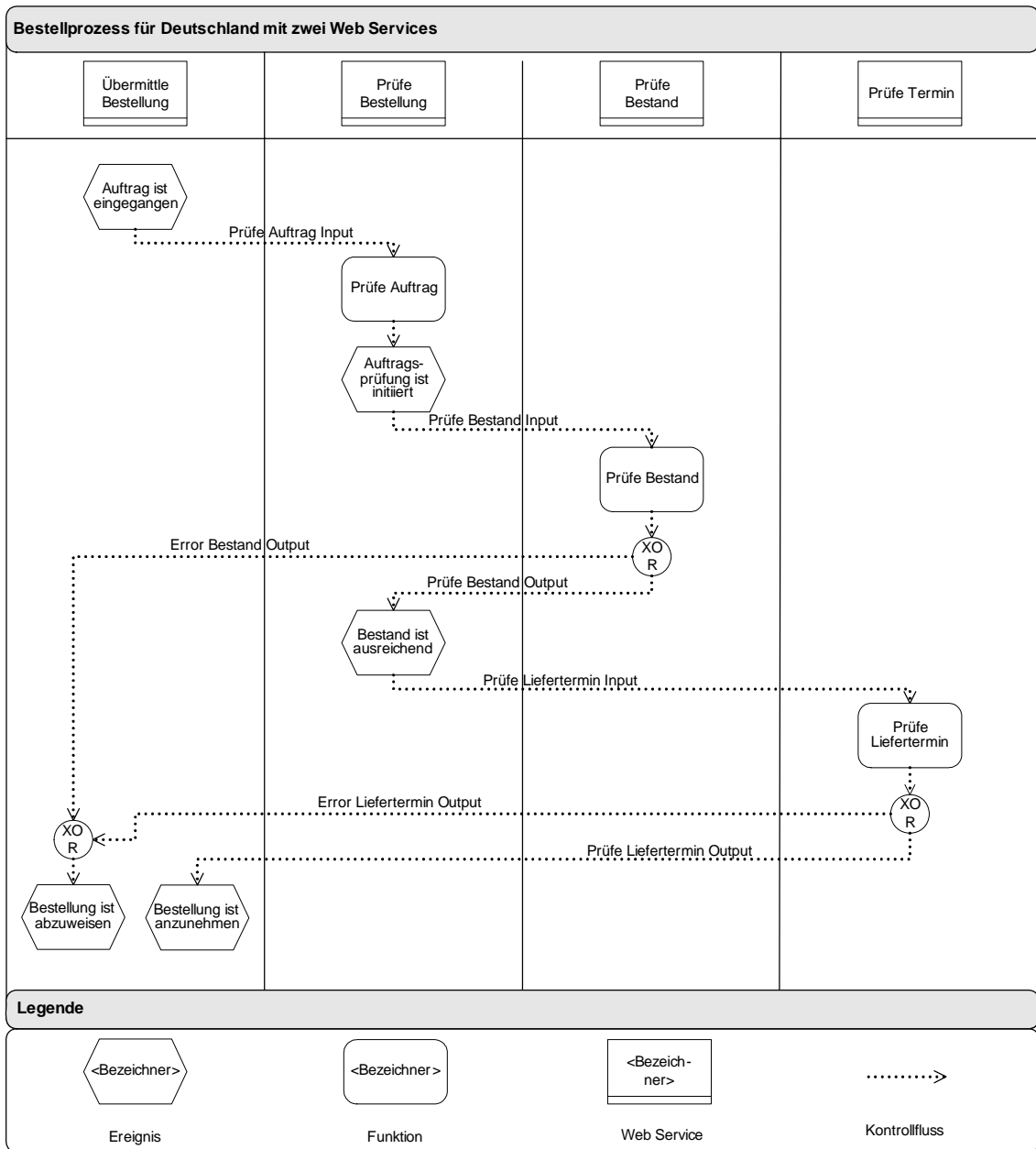
Abbildung 33: Darstellung der Web Service-Interaktionen als eEPK
