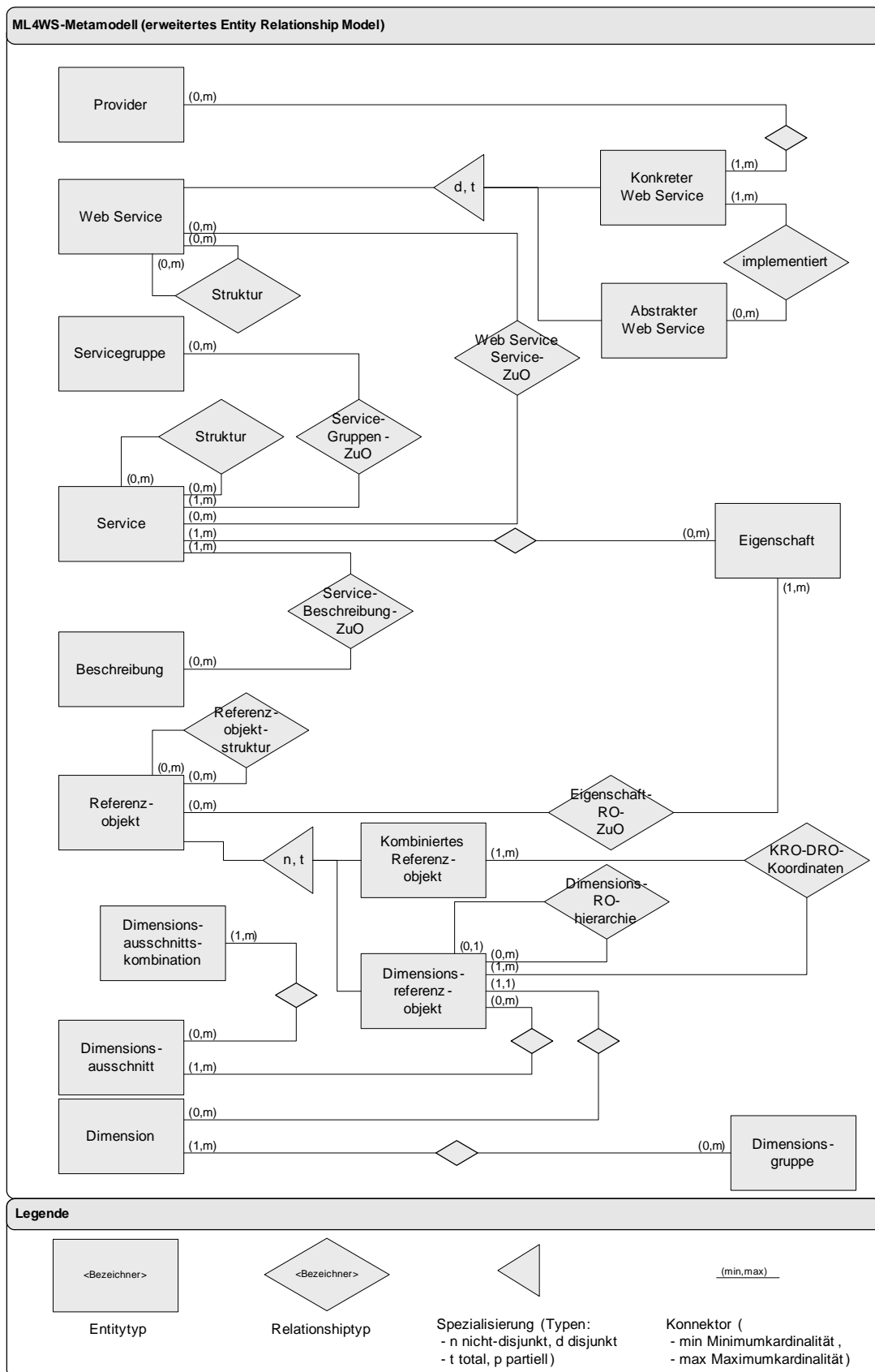
Abbildung 9: ML4WS-Matemodell des Fachkonzepts
