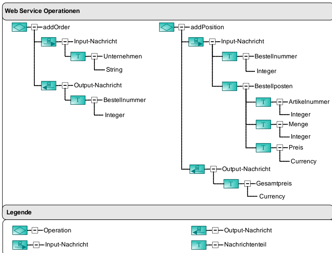
Abbildung 28: Aufgliedern eines Web Services in Operationen
