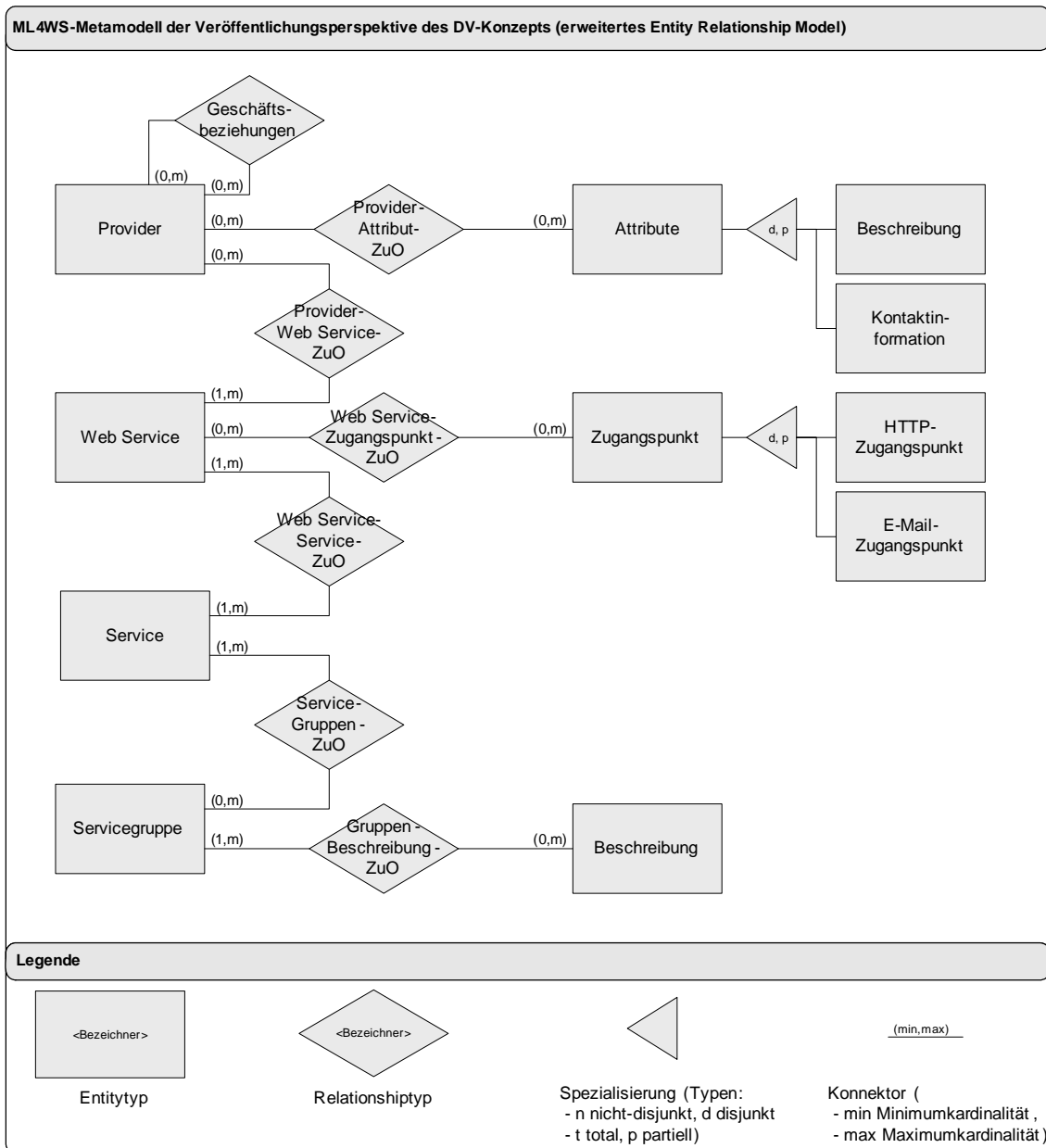
Abbildung 15: ML4WS-Metamodell der Veröffentlichungsperspektive des DV-Konzepts
