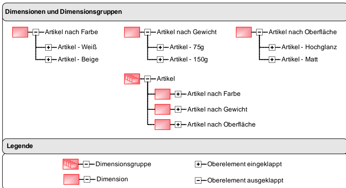
Abbildung 20: Definition der relevanten Dimensionen und Dimensionsgruppen
