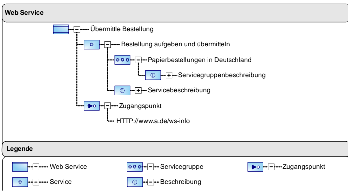
Abbildung 31: Definition eines Web Services im DV-Konzept
