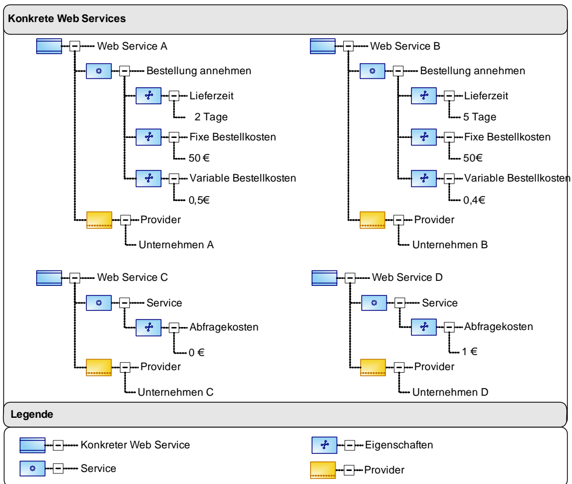
Abbildung 26: Alternative konkrete Web Services
