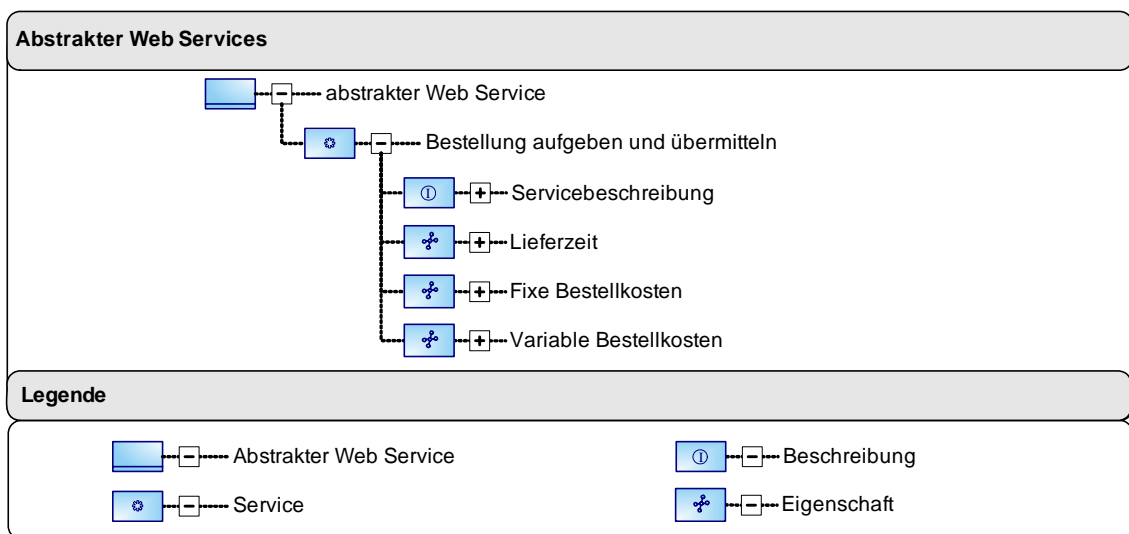
Abbildung 23: Definition eines abstrakten Web Services
