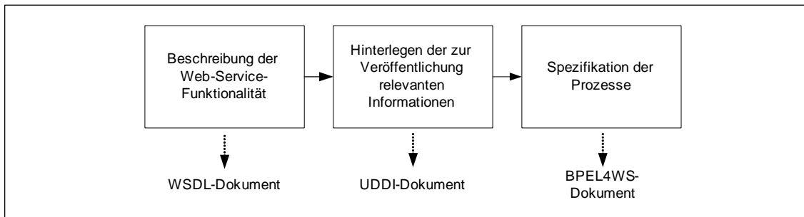
Abbildung 17: Vorgehensmodell für die Erstellung eines DV-Konzepts
