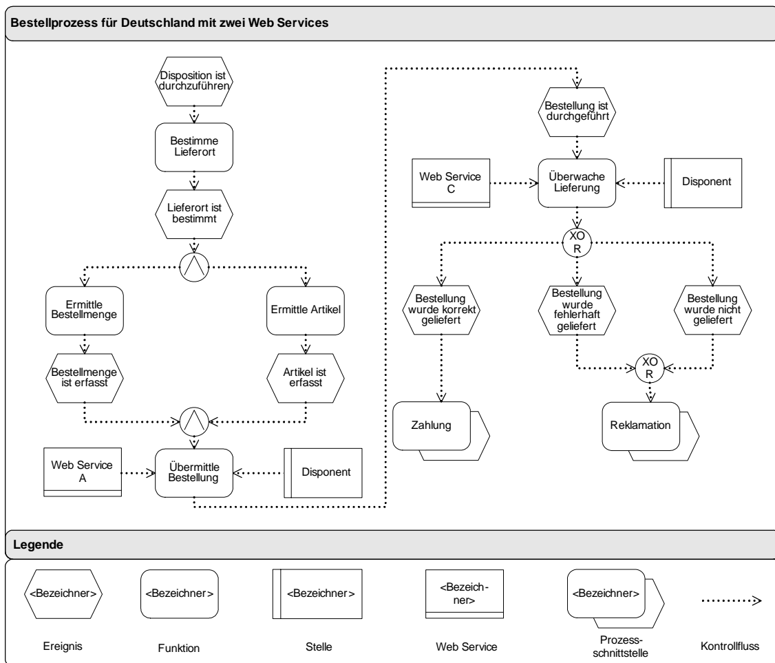
Abbildung 27: Resultierender Prozess unter Berücksichtigung der Zielsetzung
