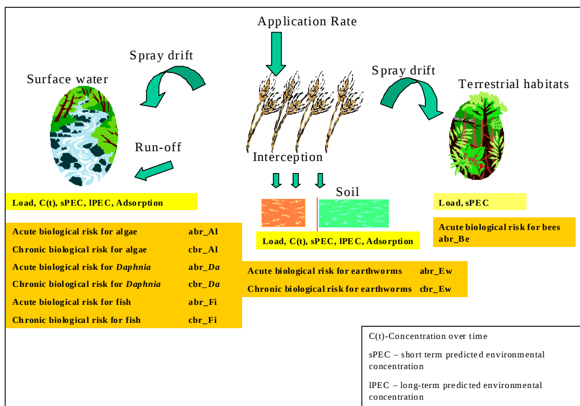
Abb. 2: Struktur des Risiko-Bewertungsmodells SYNOPS
