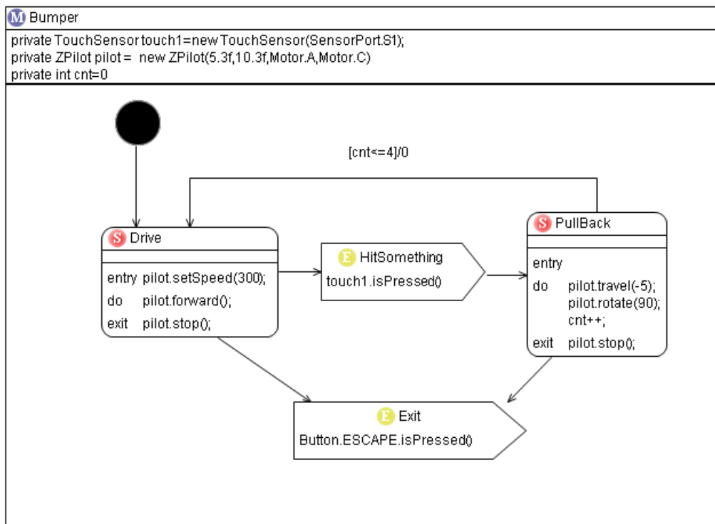
Abbildung 2.9: Das fertige Bumper Car
