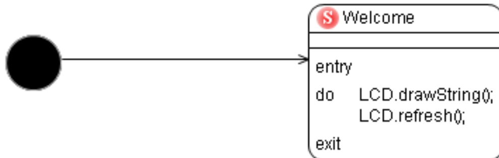
Abbildung 2.4: Einfacher Automat mit einem Zustand.
