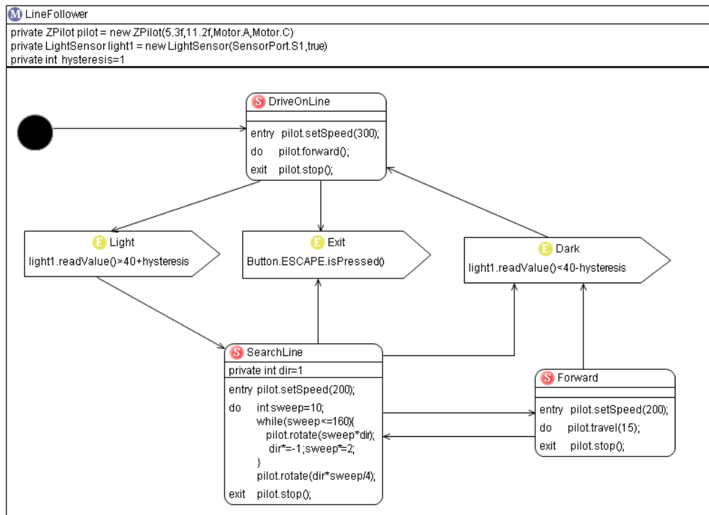
Abbildung 2.10: Fährt auf unterbrochenen Linien
