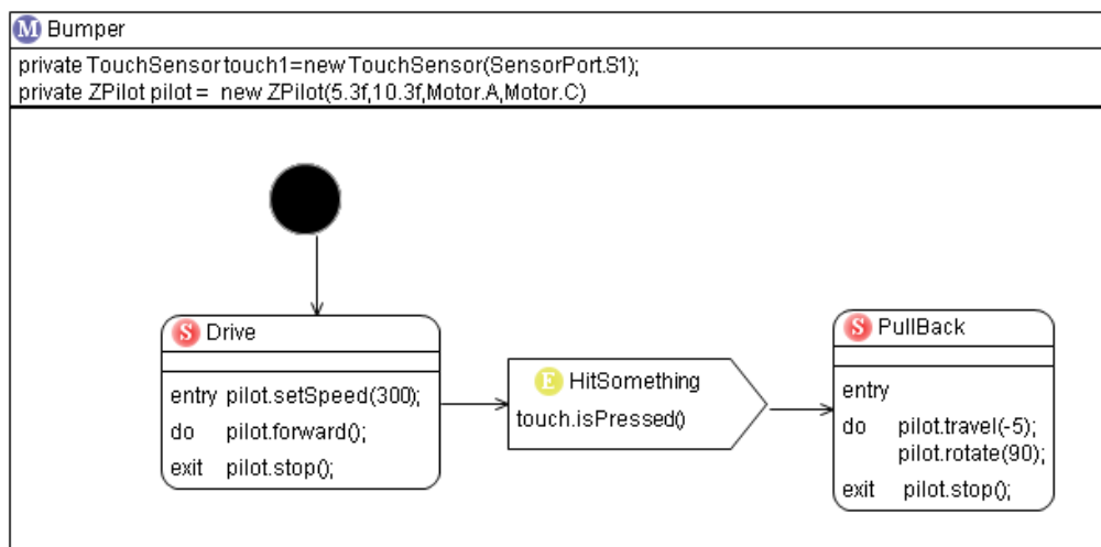
Abbildung 2.8: Durch Touch Sensor ausgelöstes Event
