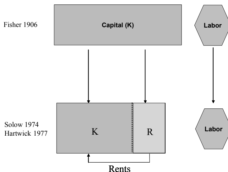
Abb. 1: Kapital in Solow's Wachstumsmodell
