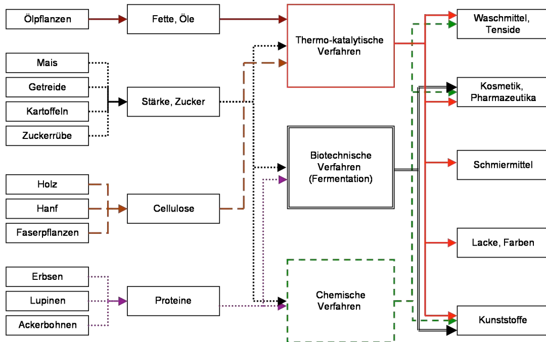
Abbildung 2.1: Überblick über exemplarische Nawaro-Pfade zur stofflichen Nutzung (eigene Darstellung)
