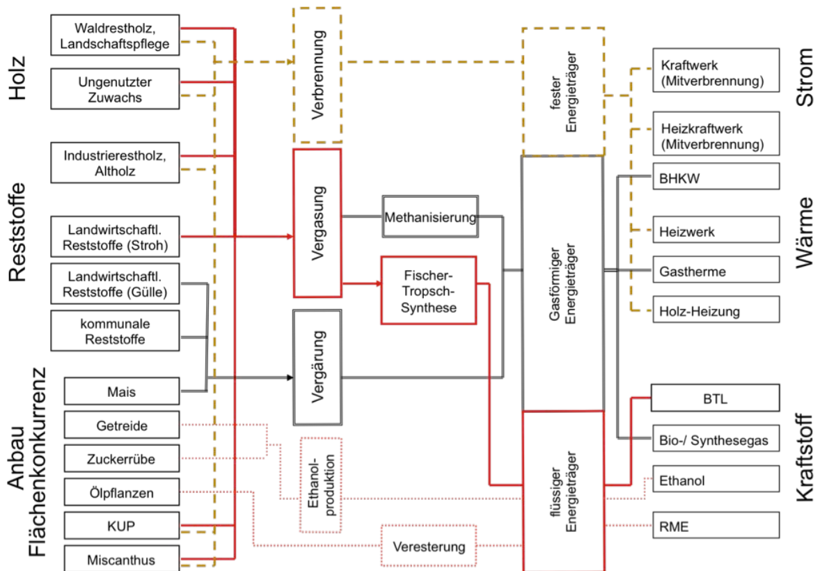
Abbildung 2.2: Überblick über exemplarische Nawaro-Pfade zur energetischen Nutzung (eigene Darstellung)
