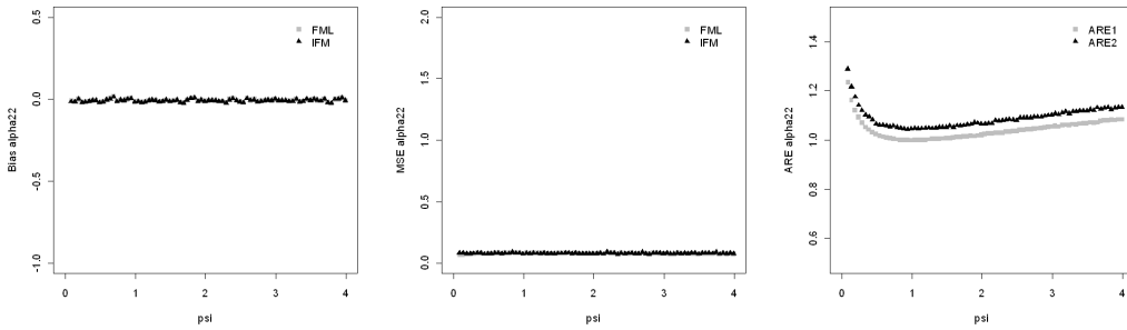
Abbildung 15: Ergebnis Szenario (3) für den Parameter \alpha_{22} mit m_j = 3 , \alpha_j = (-0.5, 0.5) , \beta_j = 0.5 , n = 100 , k = 1000 und 0 < \psi \leq 4
