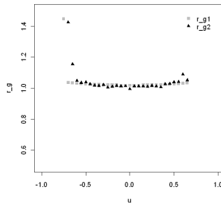
Abbildung 27: Verallgemeinerte Effizienzverhältnis r_g Szenario (2b) mit m_j = 3 , \alpha_j = (-0.5, 0.5) , \beta_j = 0.5 , \psi = 4 , n = 100 , k = 1000 und -0.8 \leq u_j \leq 0.8
