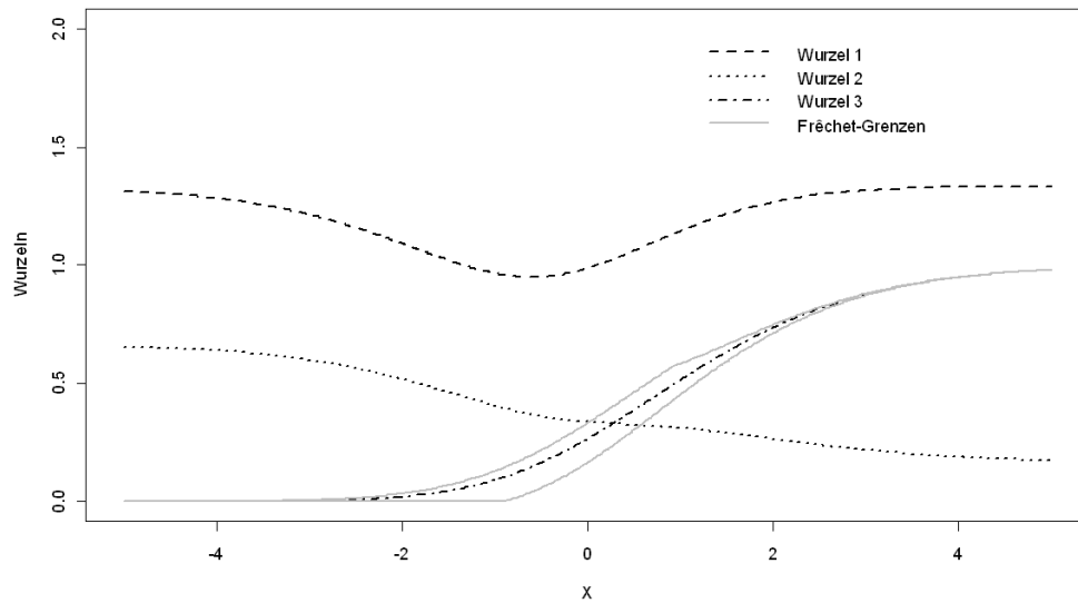
Abbildung 1: Lösungen des Polynom 4. Grades mit der Plackett-Copula
