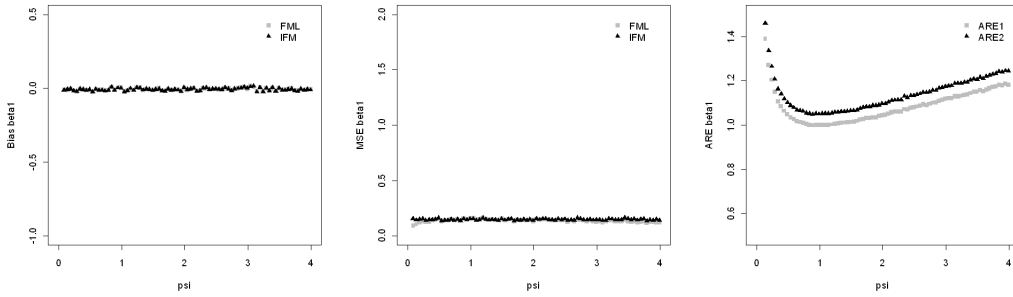
Abbildung 13: Ergebnis Szenario (3) für den Parameter \beta_1 mit m_j = 3 , \alpha_j = (-0.5, 0.5) , \beta_j = 0.5 , n = 100 , k = 1000 und 0 < \psi \leq 4
