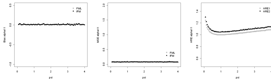
Abbildung 11: Ergebnis Szenario (3) für den Parameter \alpha_{11} mit m_j = 3 , \alpha_j = (-0.5, 0.5) , \beta_j = 0.5 , n = 100 , k = 1000 und 0 < \psi \leq 4
