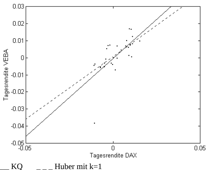
Abb. 3: Die Entstehung der KQ- und M-Regressionsgerade von VEBA am Tag 1681
