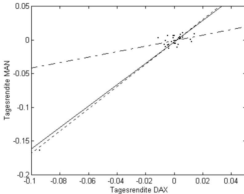
Abb. 5: Die Entstehung der KQ-, M- und GM-Regressionsgerade der MAN am Tag 739
