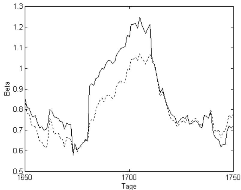
Abb. 4: Die 30-Tages-Betafaktoren von VEBA von Tag 1650 bis 1750
