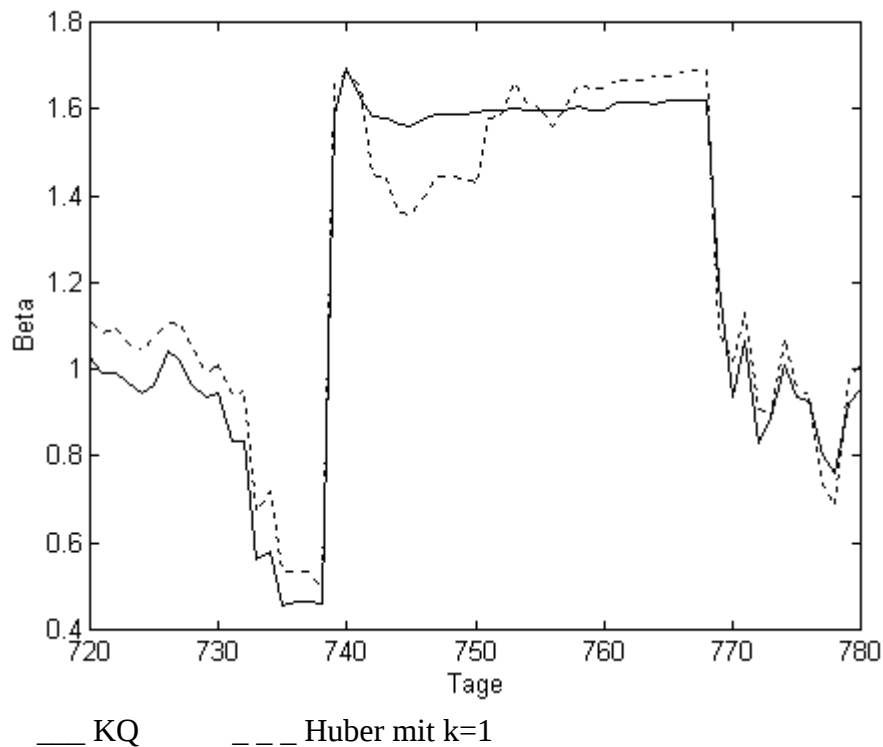
Abb. 6: Die 30-Tages-Betafaktoren der MAN von Tag 720 bis 780
