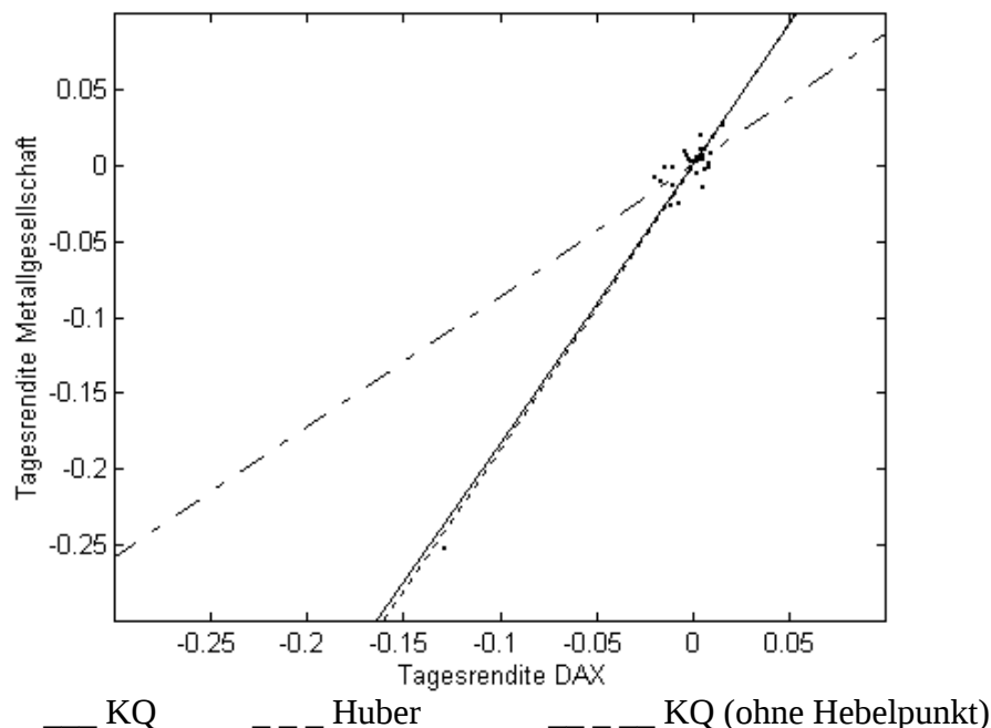
Abb.9: Die Entstehung der KQ- und M-Regressionsschätzung der Metallgesellschaft am Tag 113
