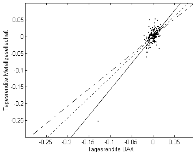
Abb.8: Die Entstehung der KQ- und M-Regressionsgerade der Metallgesellschaft am Tag 113
