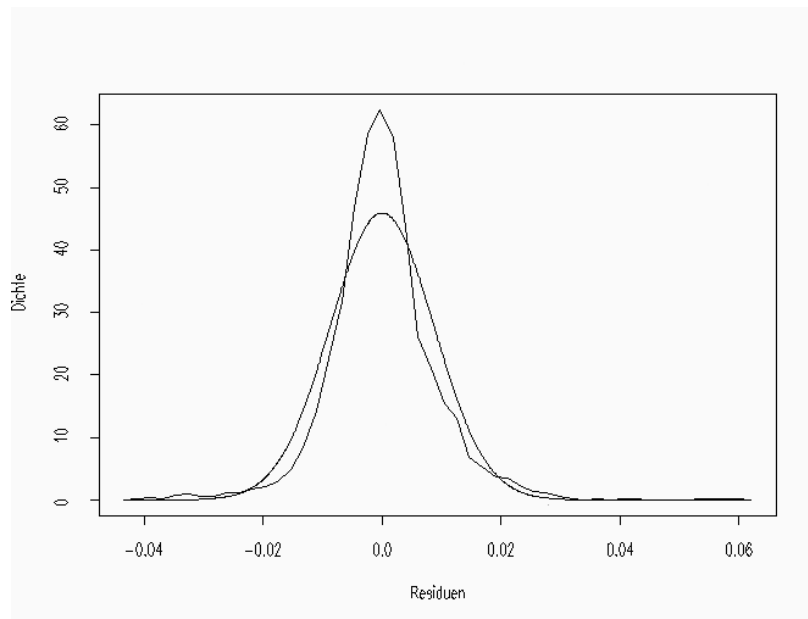
Abb. 1: Nichtparametrische Dichteschätzung der Residuen
