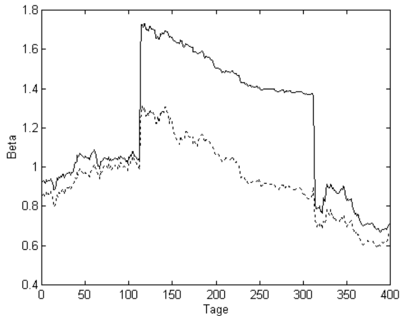
Abb. 7: Die 30-Tages-Betafaktoren der Metallgesellschaft von Tag 1 bis 400
