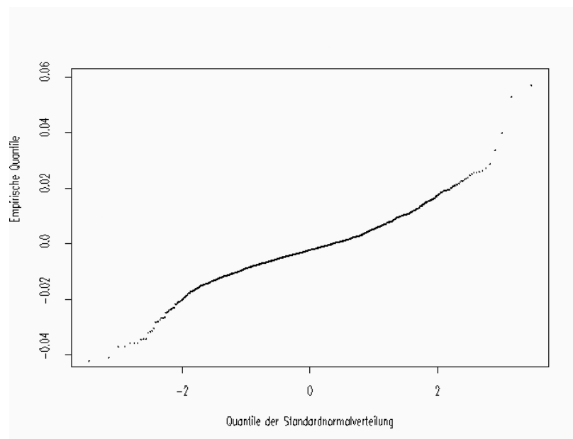
Abb. 2: QQ-Plot der Residuen und der Standardnormalverteilung
