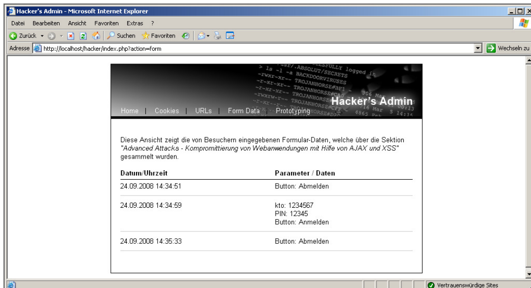
Abbildung 6: Das Angreifer-Tool
