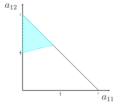
Feasible set \mathcal{S}_6
