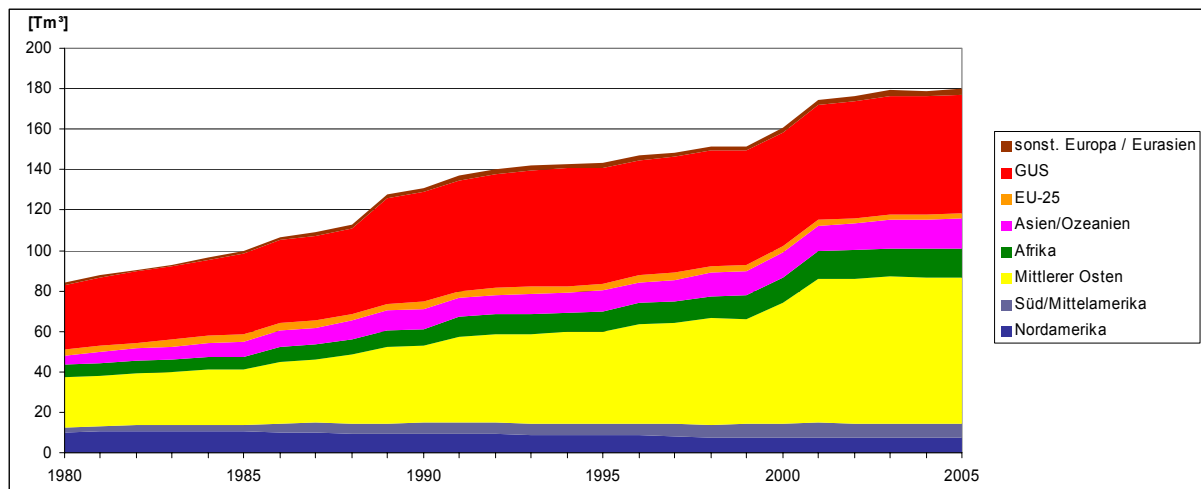
Abbildung 2: Entwicklung der weltweiten Erdgasreserven
