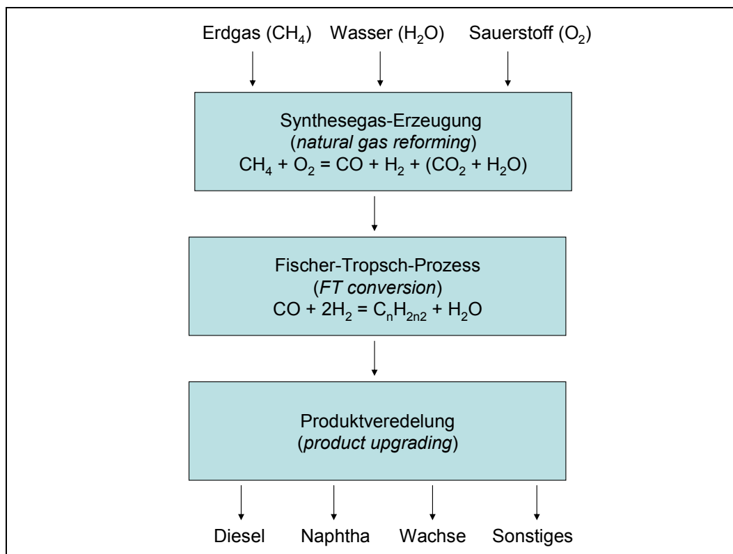
Abbildung 5: Fischer-Tropsch-Prozess 24
