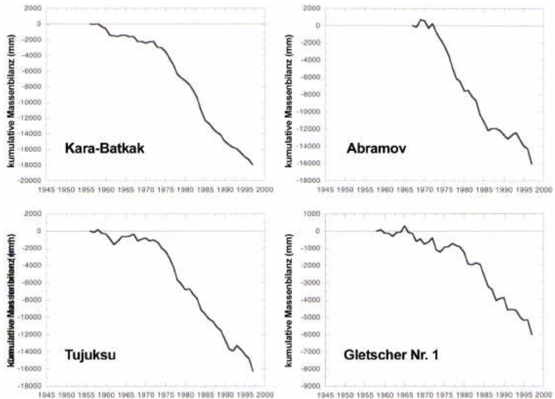
Abb. 5: Kumulative Massenbilanzkurven von Gletschern aus dem Tjan'-Šan' und dem Alaj (Quelle: WGMS 1999). 1 – Kara-Batkak (Terskej Alatau), 2- Abramov (Alaj), 3 – Zentraler Tjuksu (Zailiskij Alatau), 4 – Gletscher Nr. 1 (Tianger).
