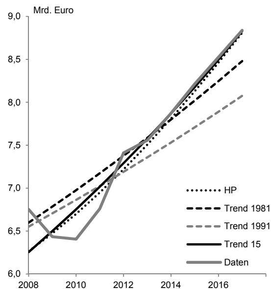
Abbildung 10: Steuereinnahmetrend aus der Sicht Mai 2013 (Variante II)
