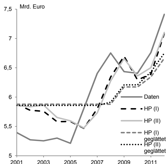
Abbildung 14: Ergebnisse des Echtzeittrendglätters für den HP-Filter 2001–2011
