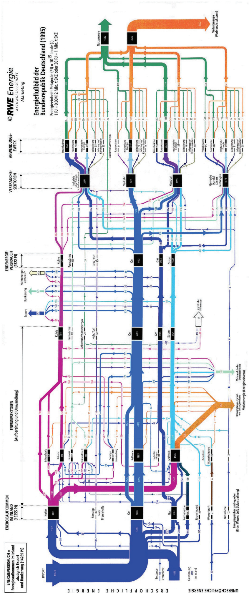
Abb. 2: Energieflussbild Deutschland zum Jahr 1995. Die Angaben sind in Petajoule. Quelle: RWE.
