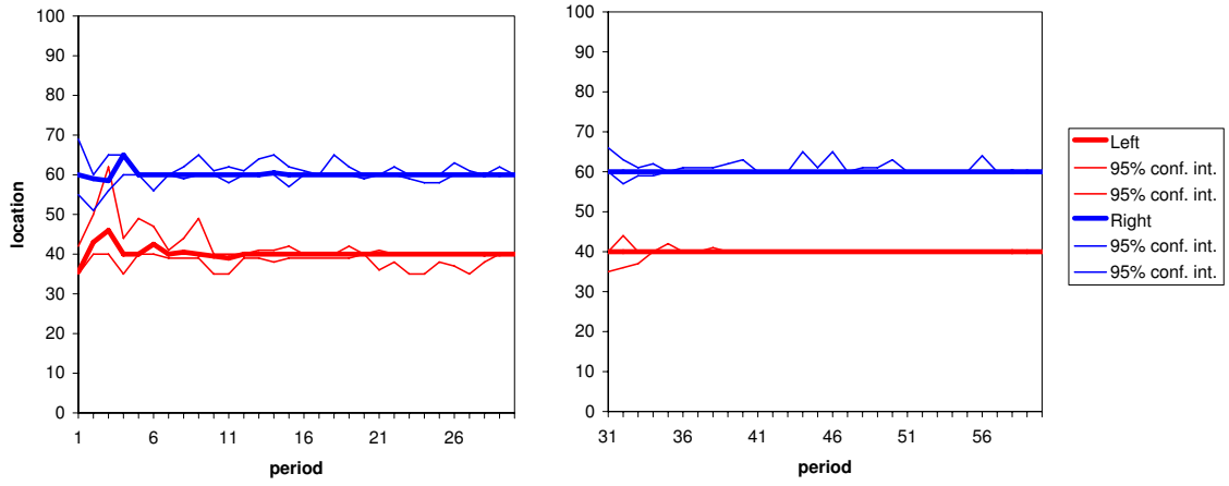
(d) Treatment 4: x_L^* = 40 & x_R^* = 60 .
