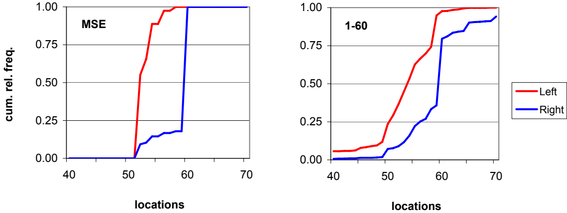
(d) Cumulative relative frequencies.
