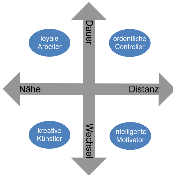
Abbildung 4.5: Riemann-Thomann-Modell 72
