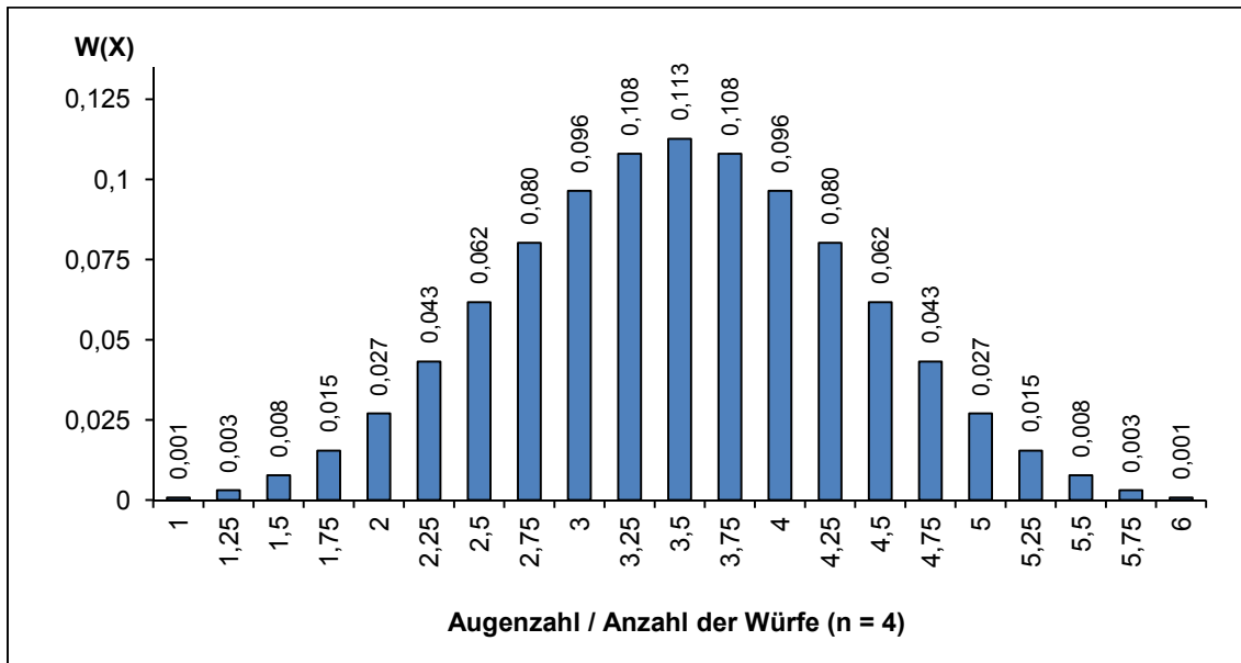
Abb. 4: Wahrscheinlichkeiten der Ereignisse bei einem viermaligen Würfelwurf
