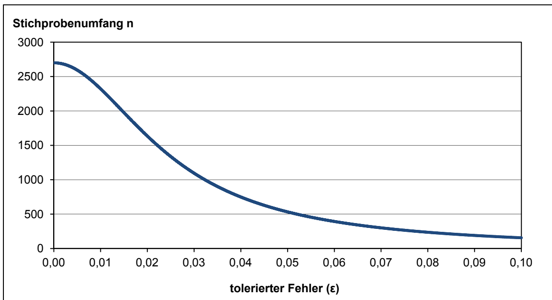
Abb. 12: Minimal erforderlicher Stichprobenumfang n in Abhängigkeit vom tolerierten Fehler \varepsilon bei konstant gewählter Grundgesamtheit N = 2700 mit einer Sicherheitswahrscheinlichkeit von 99% ( z = 2,575 )
