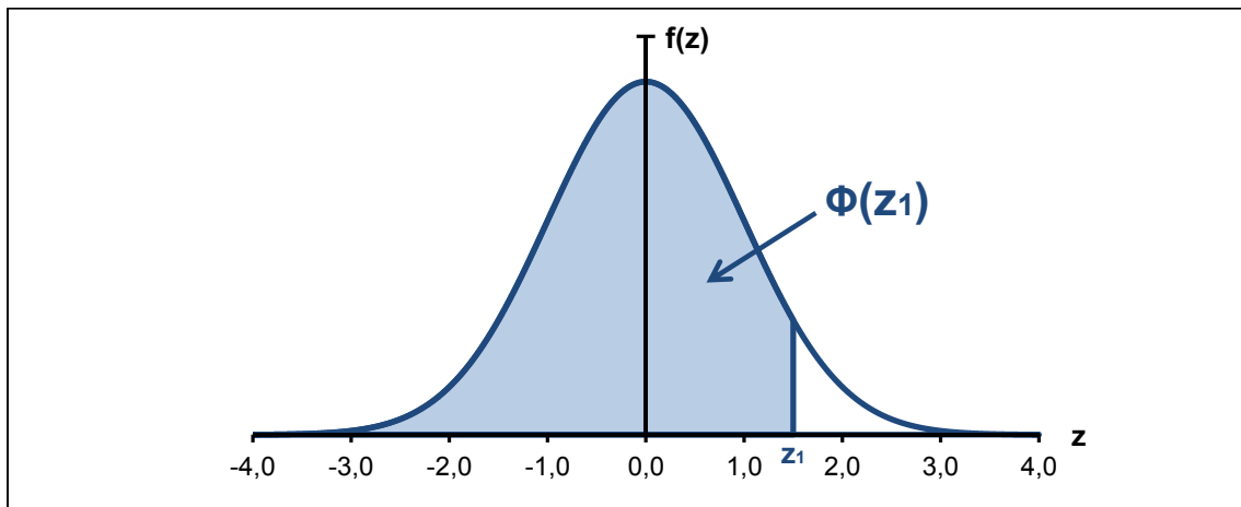
Abb. 8: Linksseitige Wahrscheinlichkeit der Standardnormalverteilung
