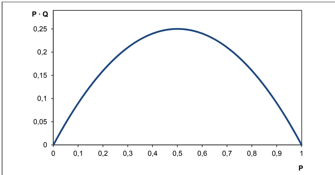
Abb. 10: Graphische Darstellung der Funktion P \cdot Q mit Q = 1 - P und 0 \leq P \leq 1 . P \cdot Q ist maximal für P=Q=0,5 .
