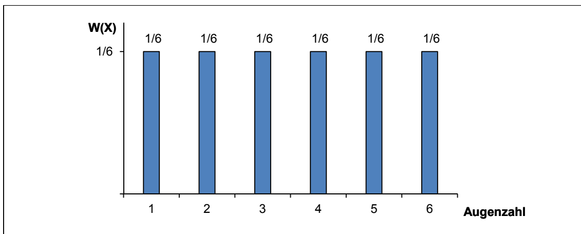
Abb. 1: Wahrscheinlichkeiten der Ereignisse beim einmaligen Würfelwurf
