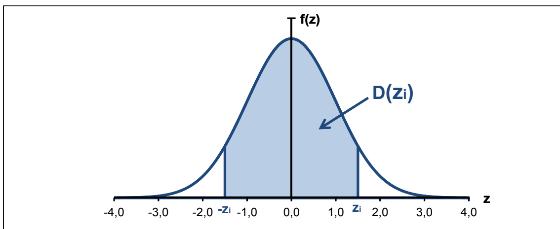
Abb. 9: Zentrale Wahrscheinlichkeit der Standardnormalverteilung
