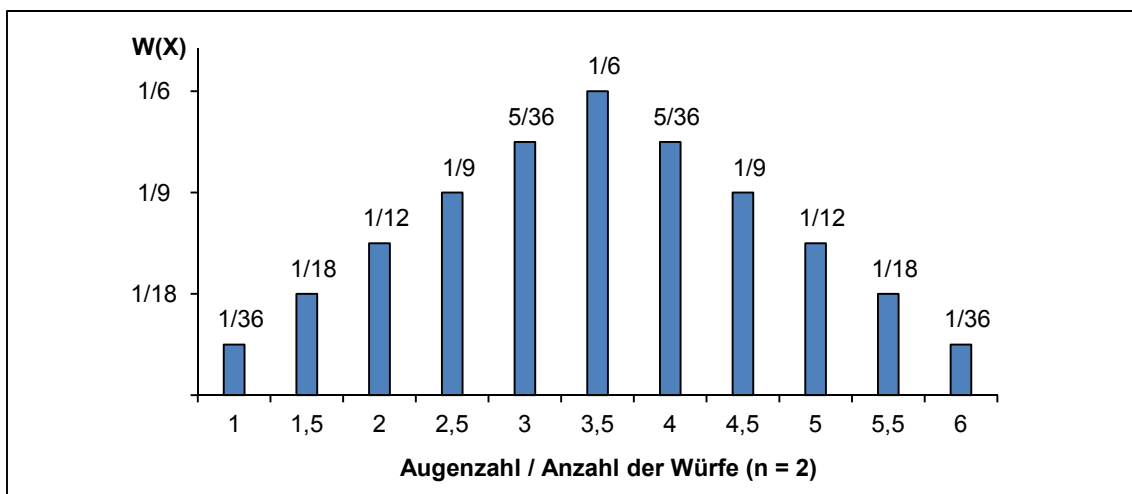
Abb. 2: Wahrscheinlichkeiten der Ereignisse bei zweimaligem Würfelwurf
