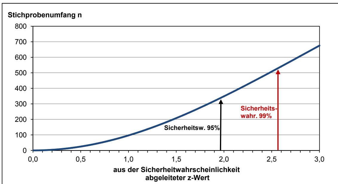
Abb. 13: Minimal erforderlicher Stichprobenumfang n in Abhängigkeit von der Sicherheitswahrscheinlichkeit bei konstanter Grundgesamtheit N = 2700 und einem konstanten tolerierten Fehler \varepsilon = 0,05 .
