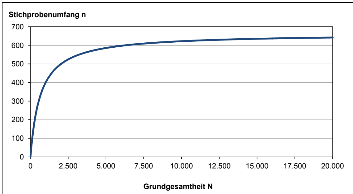
Abb. 11: Minimal erforderlicher Stichprobenumfang n in Abhängigkeit von der Grundgesamtheit N bei konstant gewählter Sicherheitswahrscheinlichkeit von 99% ( z = 2,575 ) und einem tolerierten Fehler \varepsilon = 0,05
