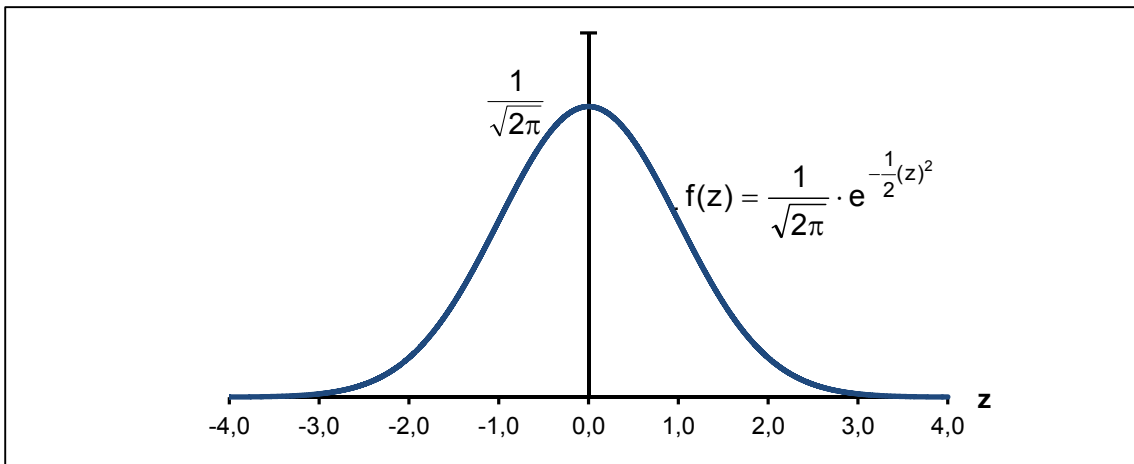
Abb. 7: Die Standardnormalverteilungsfunktion
