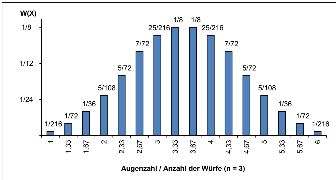
Abb. 3: Wahrscheinlichkeiten der Ereignisse bei dreifachem Würfelwurf
