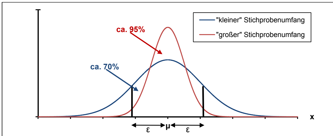
Abb. 6: Verlauf der Dichtefunktion für „kleine“ und für „große“ Stichprobenumfänge (Prozentangaben zum jeweiligen Flächeninhalt sind geschätzt)
