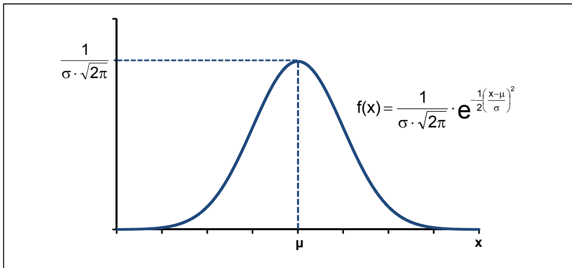
Abb. 5: Die Dichtefunktion der Normalverteilung (Gauß'sche Glockenkurve)
