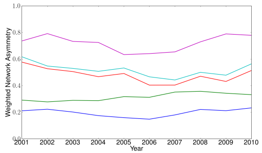
(d) Absolute weighted network asymmetry
