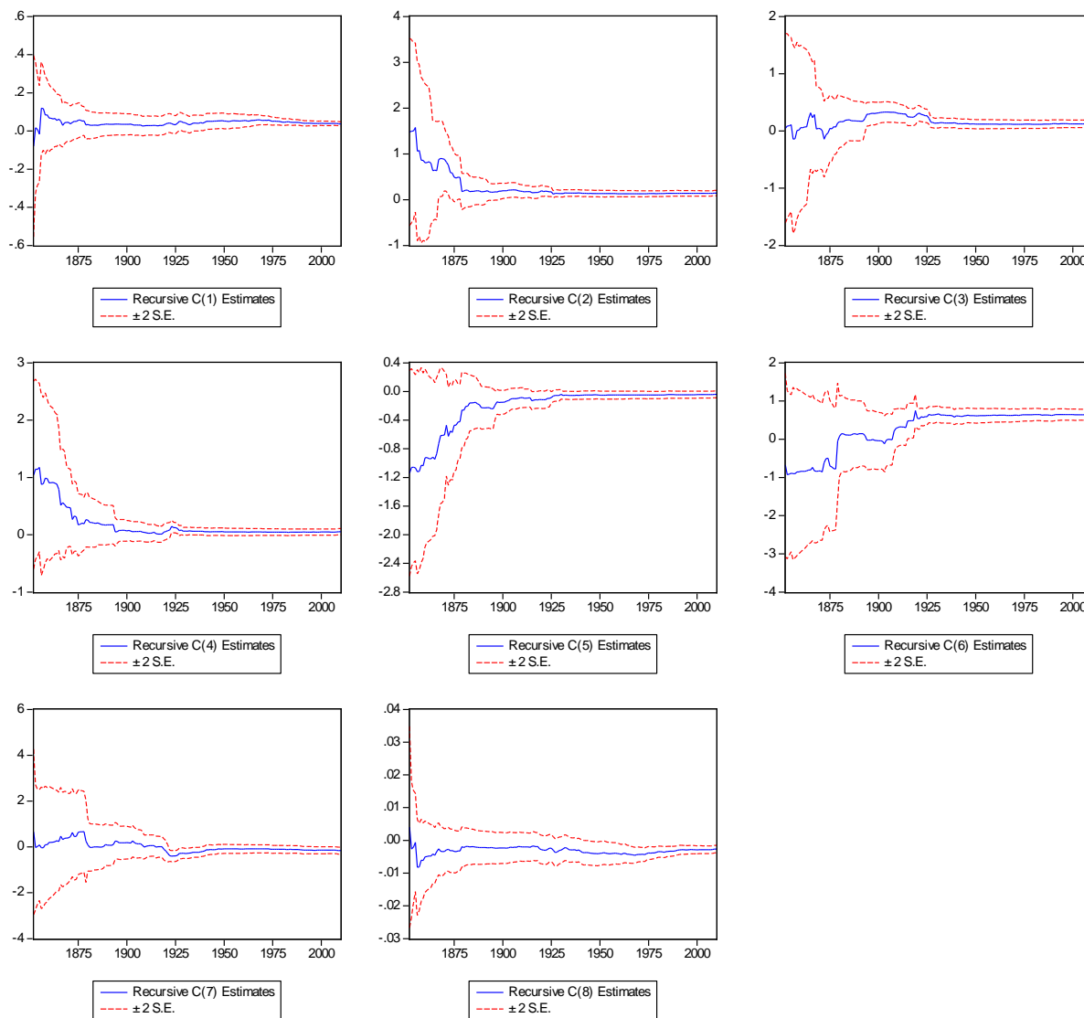
Fig. 13 RLS Parameter Plots Eq. (4): 1831-2010
