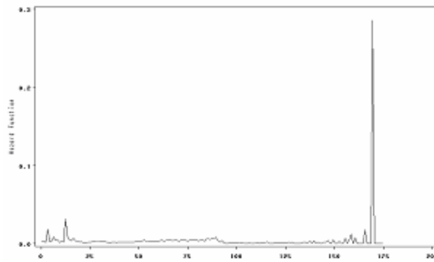
Fig. 2. Hazard function
