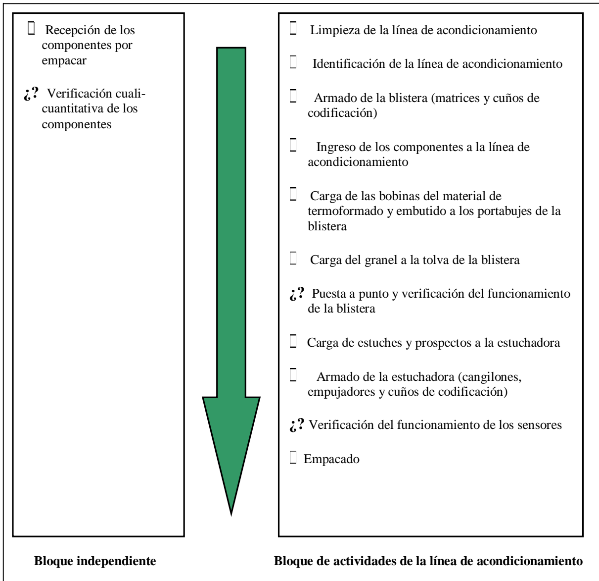
Figura 9. Diagrama de flujo del proceso de acondicionamiento.
