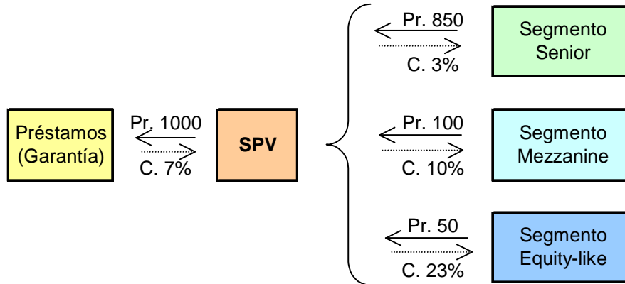
Gráfico 13: CDO tradicional*
