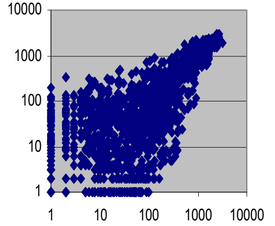
(d) \epsilon=0.02
