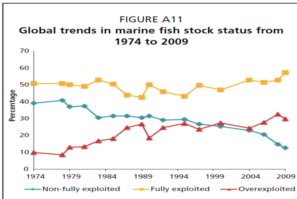
Abbildung 2-4: Entwicklung der Meeresfischbestände 1974 – 2009
