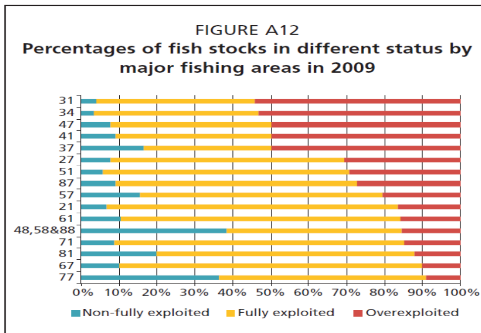
Abbildung 2-5: Anteile wenig genutzter, voll genutzter, und überfischter Bestände in verschiedenen Meeresregionen
