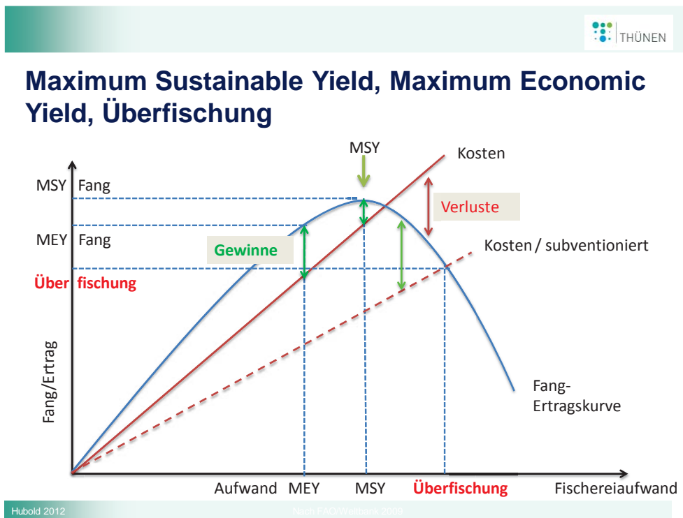
Abbildung 2-3: Überfischungskurve (nach Weltbank/FAO 2009)
