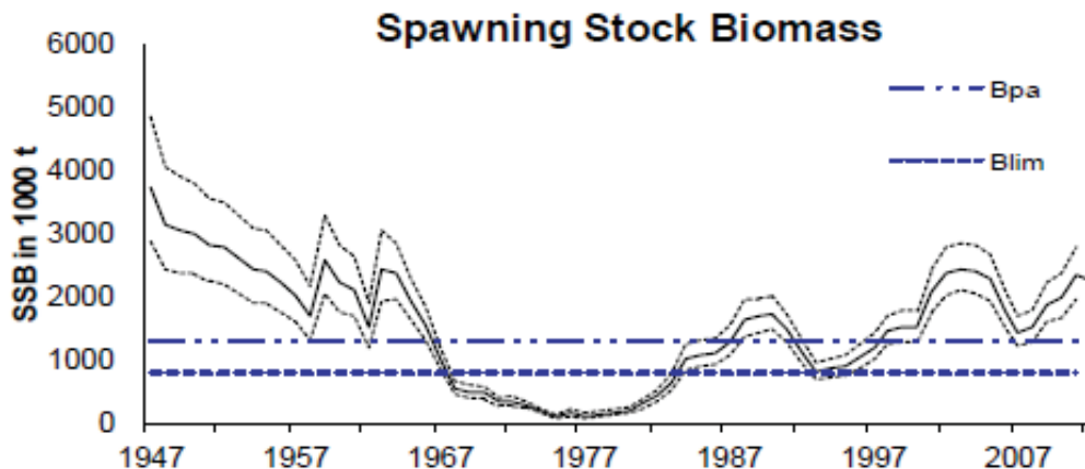
Abbildung 3-2: Entwicklung des Nordsee-Heringsbestandes
