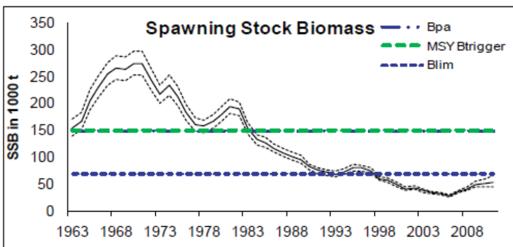
Abbildung 3-1: Entwicklung des Nordsee-Kabeljaubestandes
