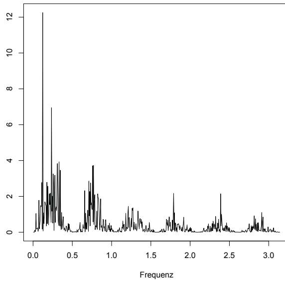
Abbildung 3: Periodogramm der Reihe \ln X_t - \ln X_{t-12} für mittlere Abflüsse am Pegel Köln
