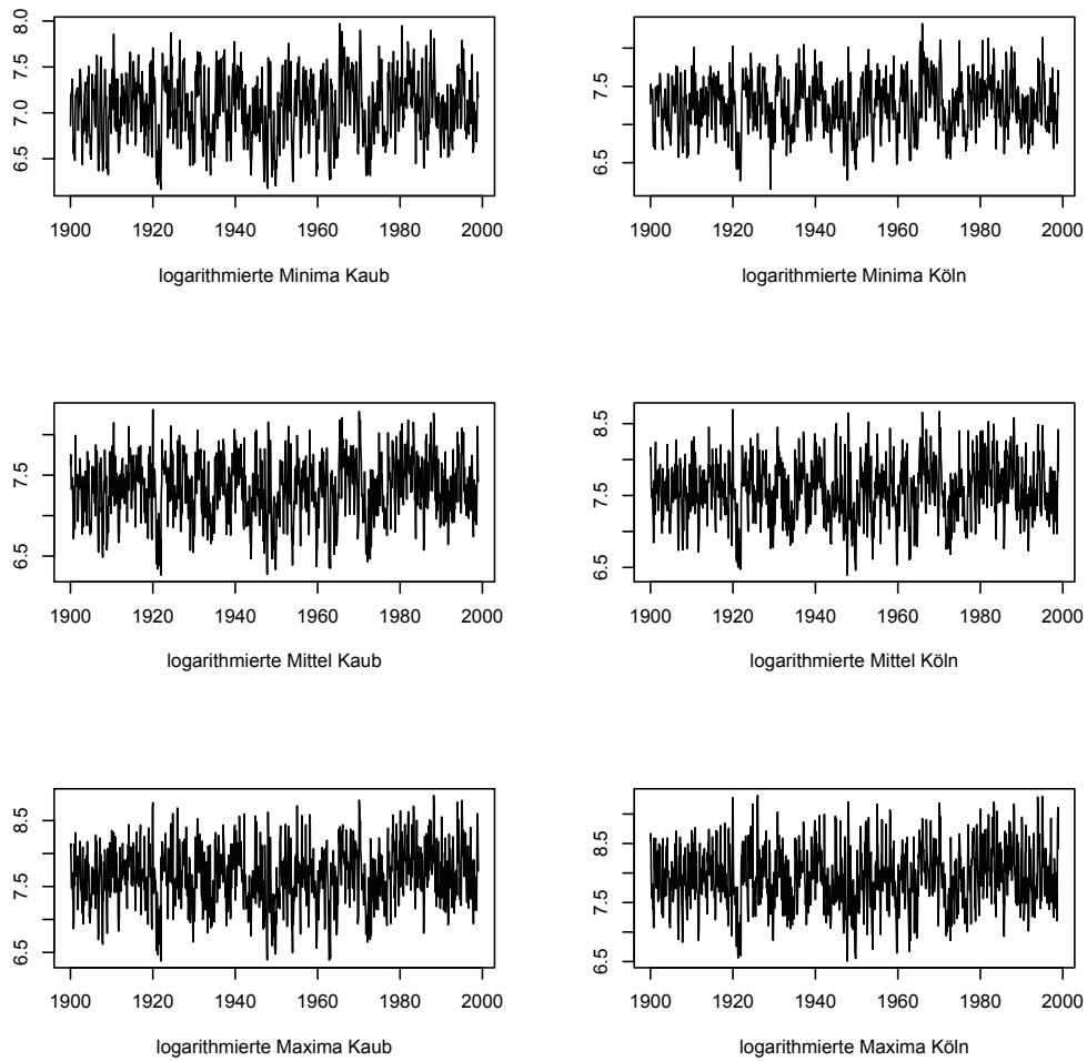
Abbildung 1: Logarithmierte Reihen des minimalen, mittleren und maximalen Abflusses am Pegel Kaub (linke Spalte) und Köln (rechte Spalte)
