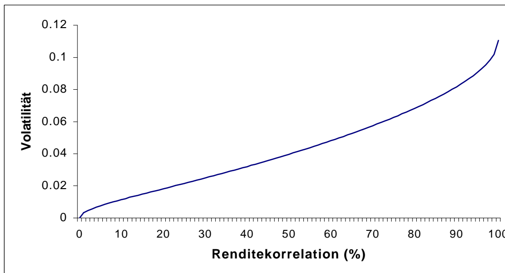
Abb. 5: Kombinationen von Renditekorrelationen und Volatilitäten mit identischer Ausfallkorrelation (mittlere Ausfallwahrscheinlichkeit 1,22%)
