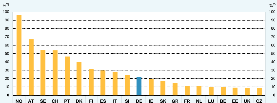
Erneuerbare Energien in ausgewählten Ländern im Jahr 2011 1)
