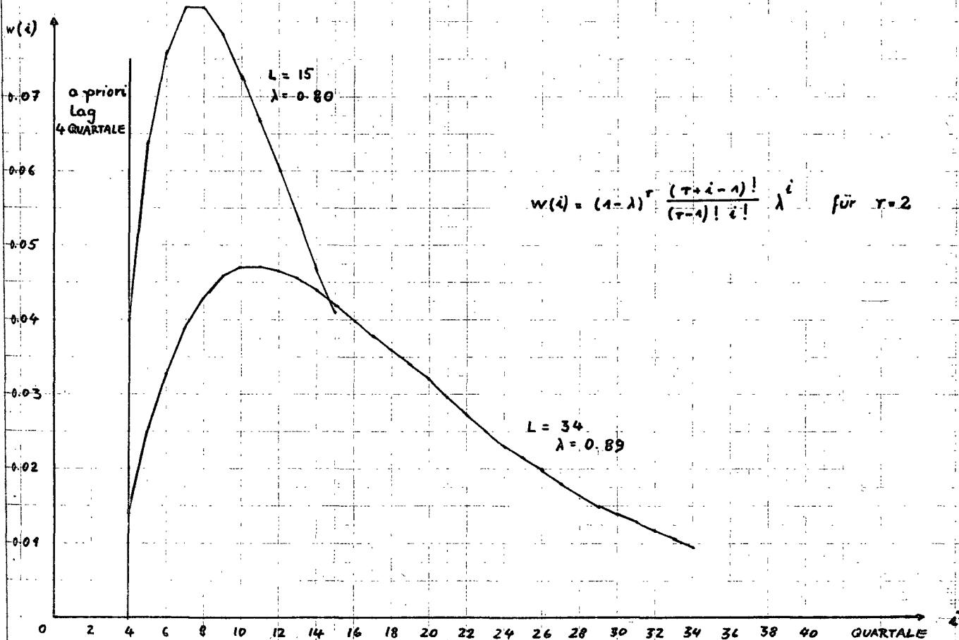
ABBILDUNG 6 VERTEILUNG DER LAG-GEWICHTE w(i) (TRUNCATED PASCAL DISTRIBUTION, R=2) ALLE BAUSPARKASSEN, GESAMTPERIODE
