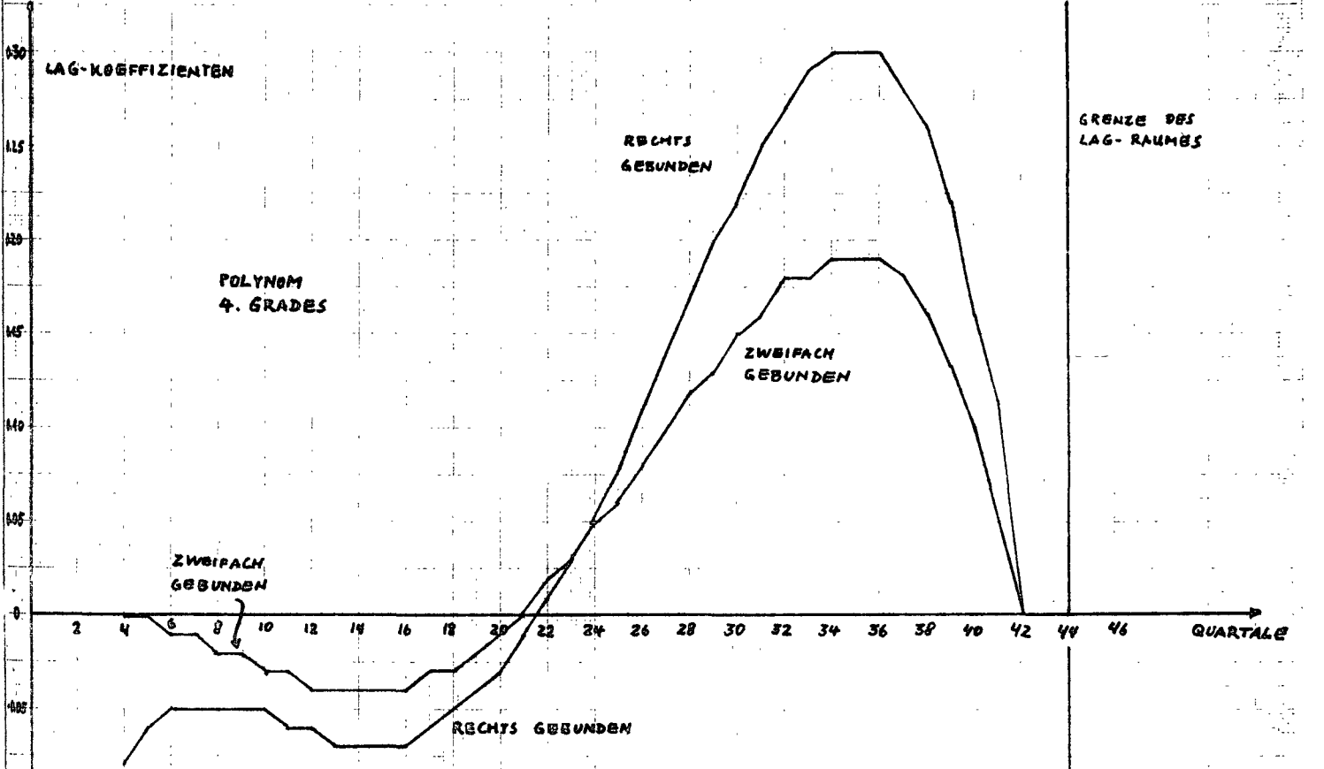
ABBILDUNG 4 VERTEILUNG DER LAG-KOEFFIZIENTEN BEI UNTERSCHIEDLICHEN BINDUNGEN (ALMON-TECHNIK, POLYNOM 4. GRADES) ALLE BAUSPARKASSEN
