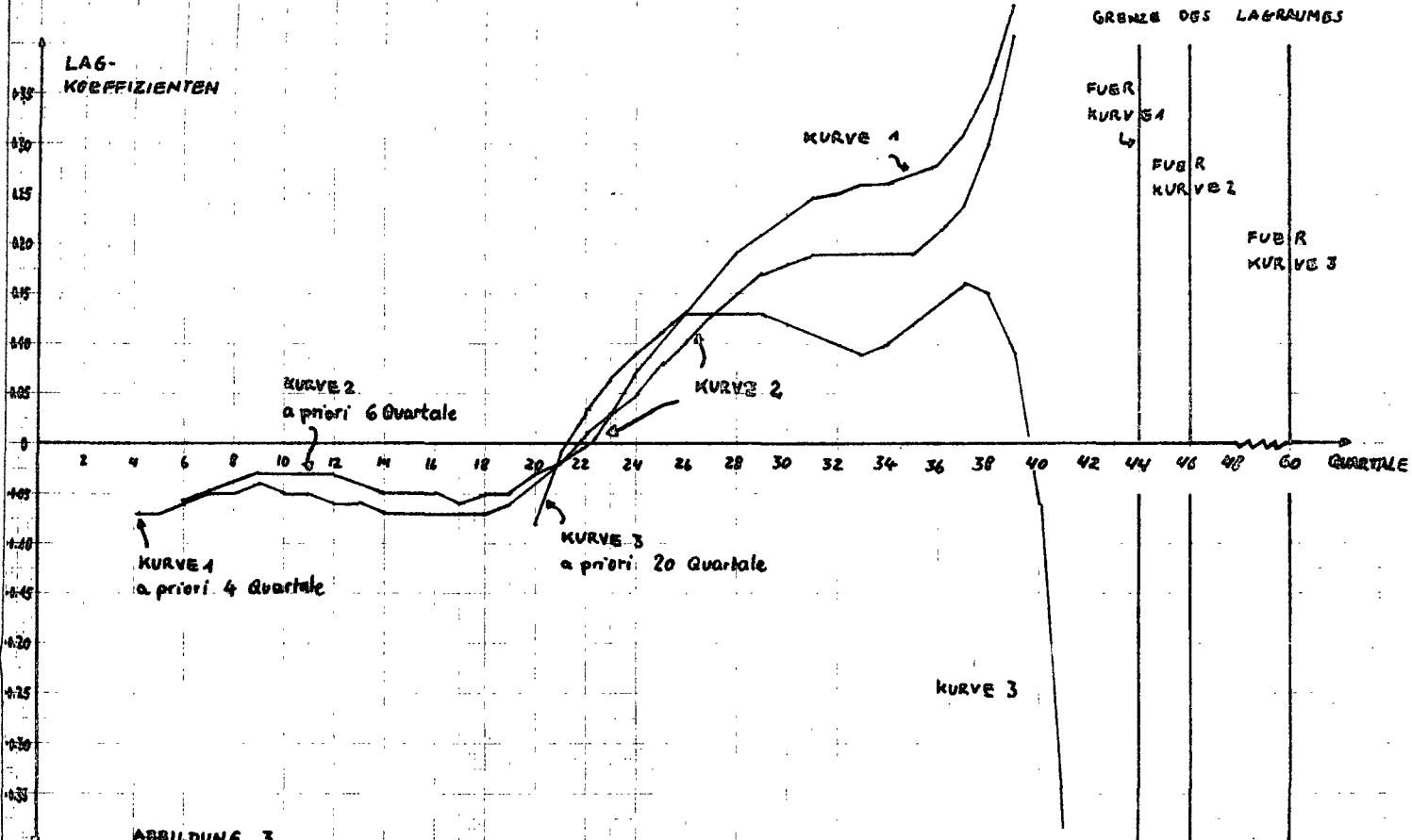
ABBILDUNG 3 VERTEILUNG DER LAG-KOEFFIZIENTEN BEIM POLYNOM 6. GRADES (ALMON-TECHNIK) ALLE BAUSPARKASSEN
