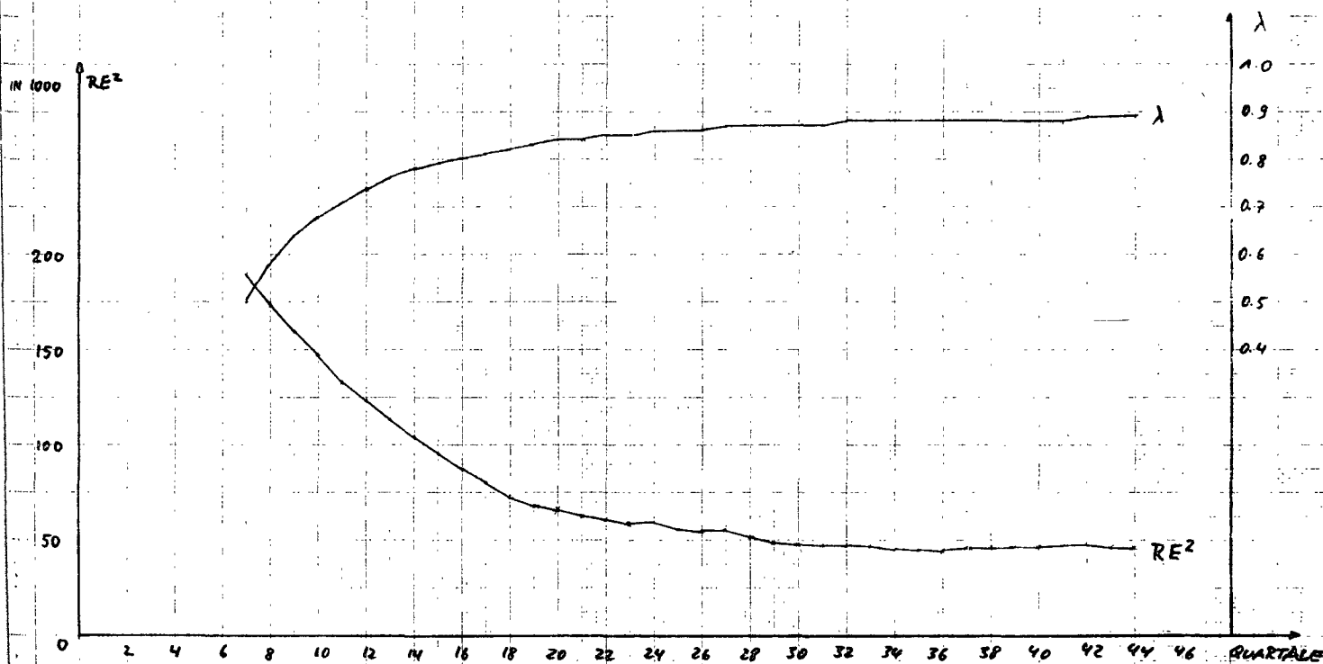
ABBILDUNG 11 DISTRIBUTED LAGS WITH TRUNCATED PASCAL DISTRIBUTION (R=2) QUADRAT DES STANDARDFEHLERS DER SCHÄTZUNG UND OPTIMALER λ-WERT ÖFFENTLICHE BAUSPARKASSEN
