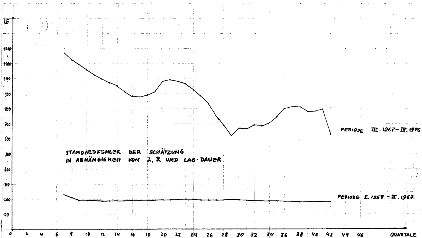
ABBILDUNG 12 DISTRIBUTED LAGS WITH TRUNCATED PASCAL DISTRIBUTION ( R=2 ) UNTERPERIODEN ALLE BAUSPARKASSEN
