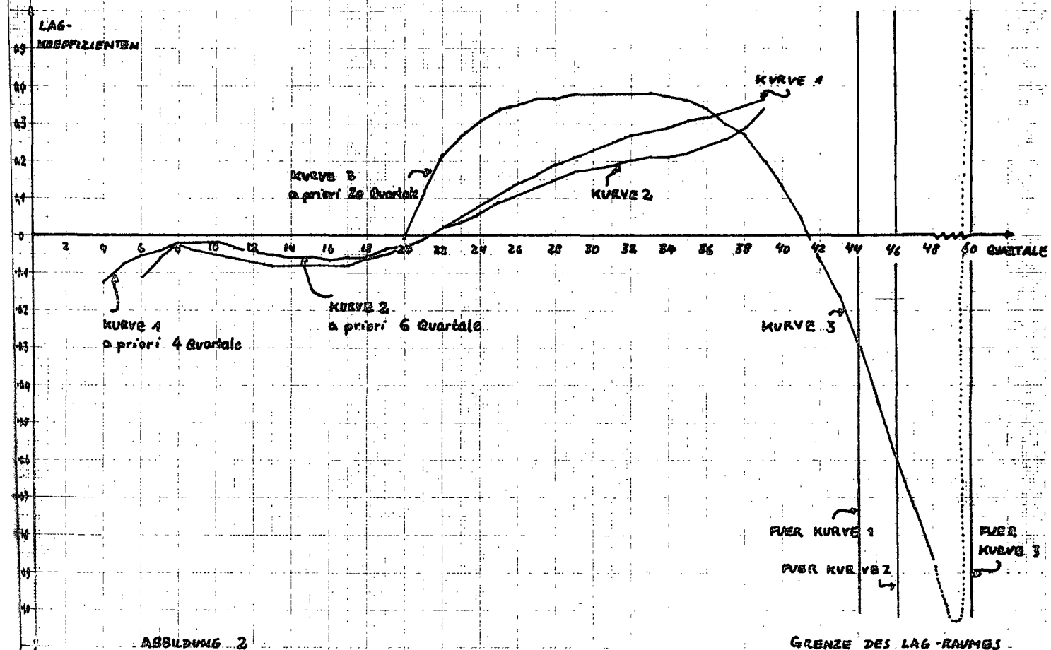
ABBILDUNG 2 VERTEILUNG DER LAG-KOEFFIZIENTEN BEIM POLYNOM 5. GRADES (ALMON-TECHNIK) ALLE BAUSPARKASSEN
