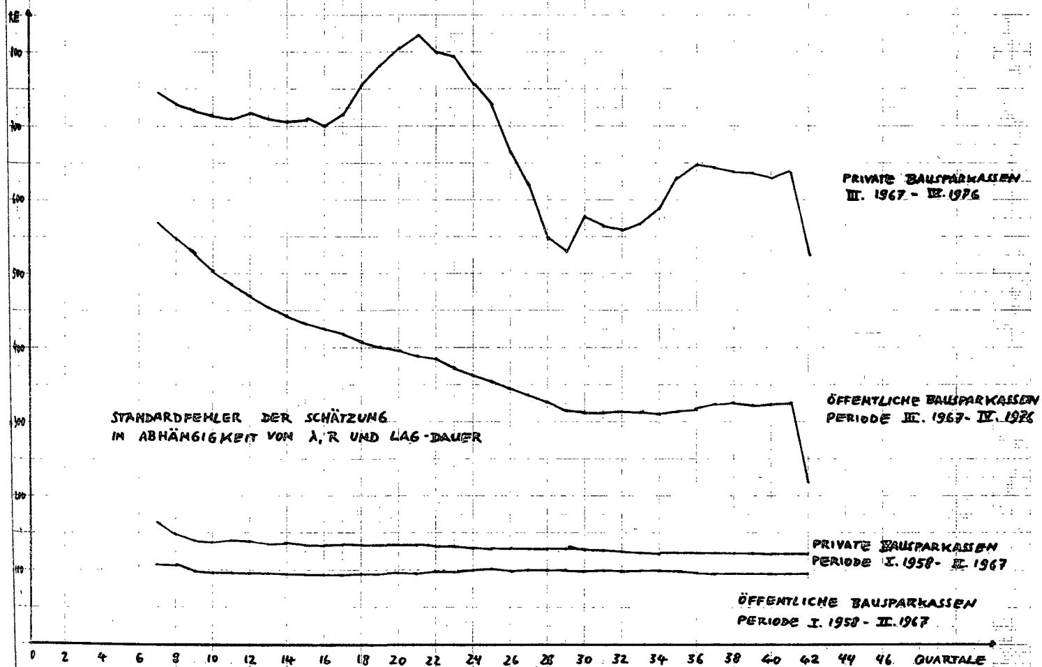
ABBILDUNG 13 DISTRIBUTED LAGS WITH TRUNCATED PASCAL DISTRIBUTION ( R=2 ) UNTERPERIODEN PRIVATE UND ÖFFENTLICHE BAUSPARKASSEN
