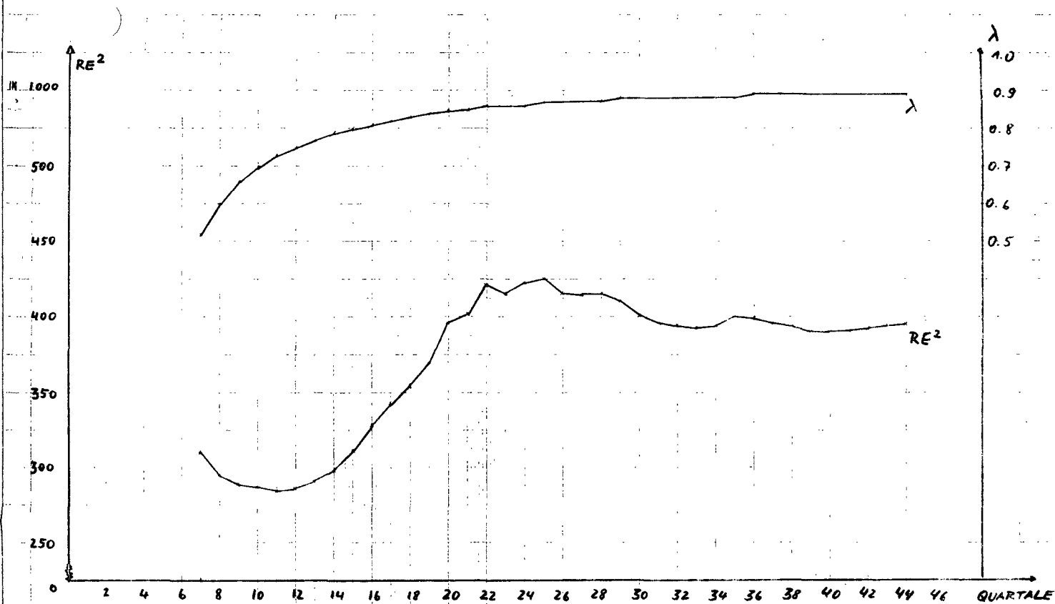
ABBILDUNG 10. DISTRIBUTED LAGS WITH TRUNCATED PASCAL DISTRIBUTION (R=2) QUADRAT DES STANDARDFEHLERS DER SCHÄTZUNG UND OPTIMALER λ-WERT PRIVATE BAUSPARKASSEN
