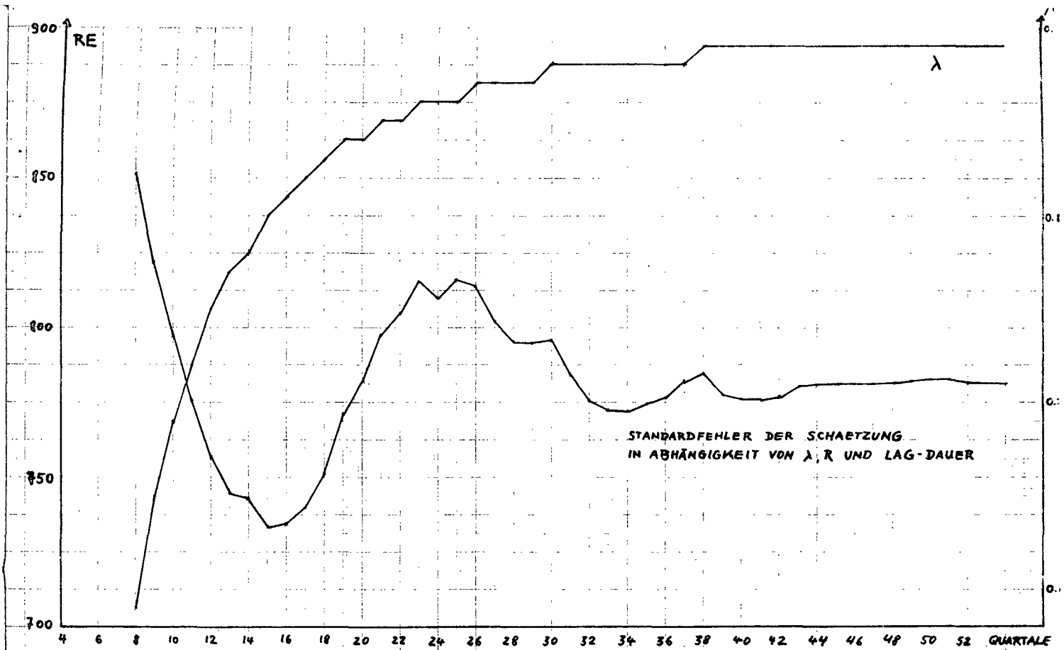
ABBILDUNG 5 DISTRIBUTED LAGS WITH TRUNCATED PASCAL DISTRIBUTION (R=2) STANDARDFEHLER DER SCHÄTZUNG UND OPTIMALER λ-WERT ALLE BAUSPARKASSEN, GESAMTPERIODE
