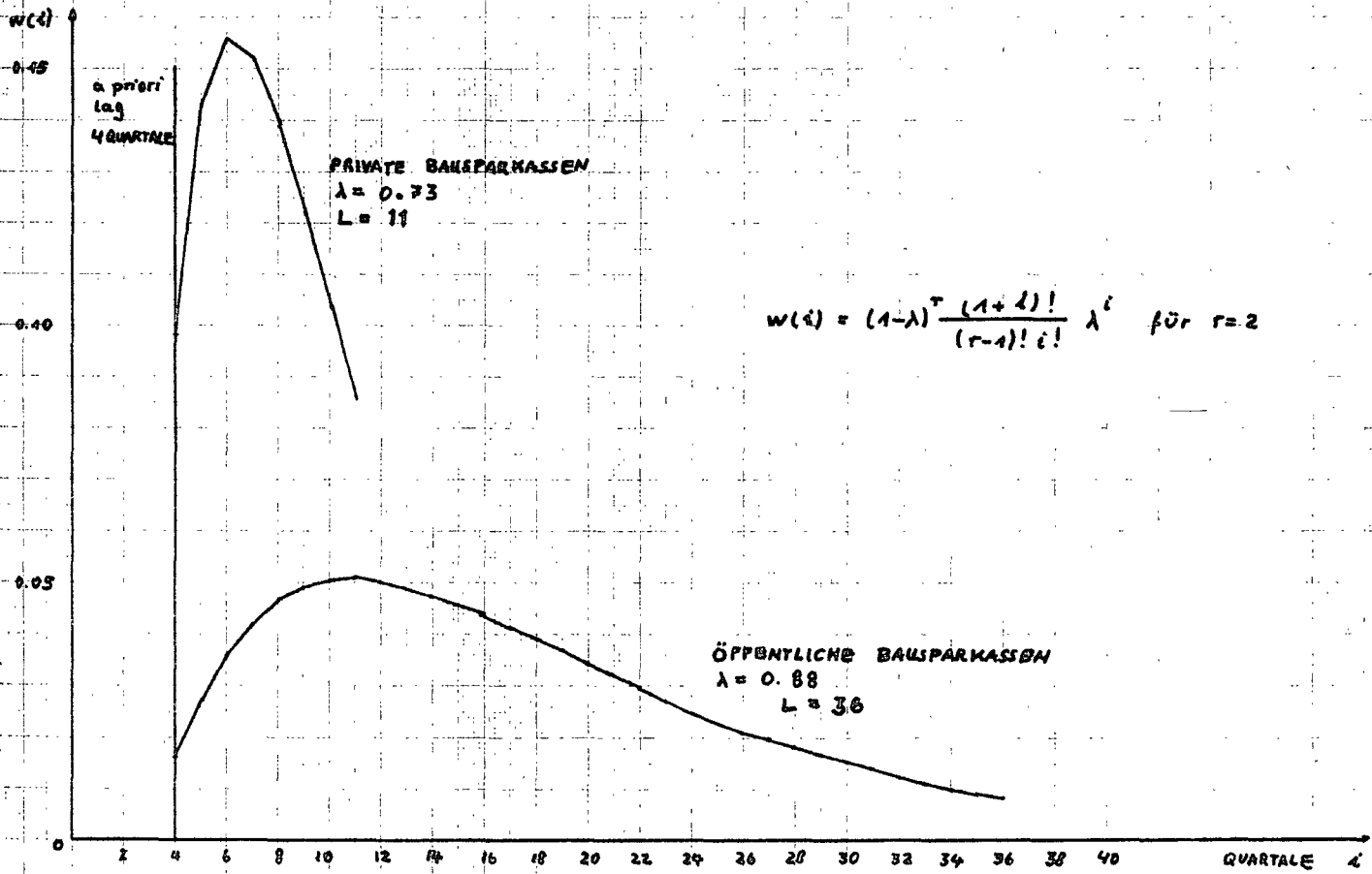
ABBILDUNG 9 VERTEILUNG DER LAG-GEWICHTE w(i) (TRUNCATED PASCAL DISTRIBUTION, R=2 ) PRIVATE UND ÖFFENTLICHE BAUSPARKASSEN
