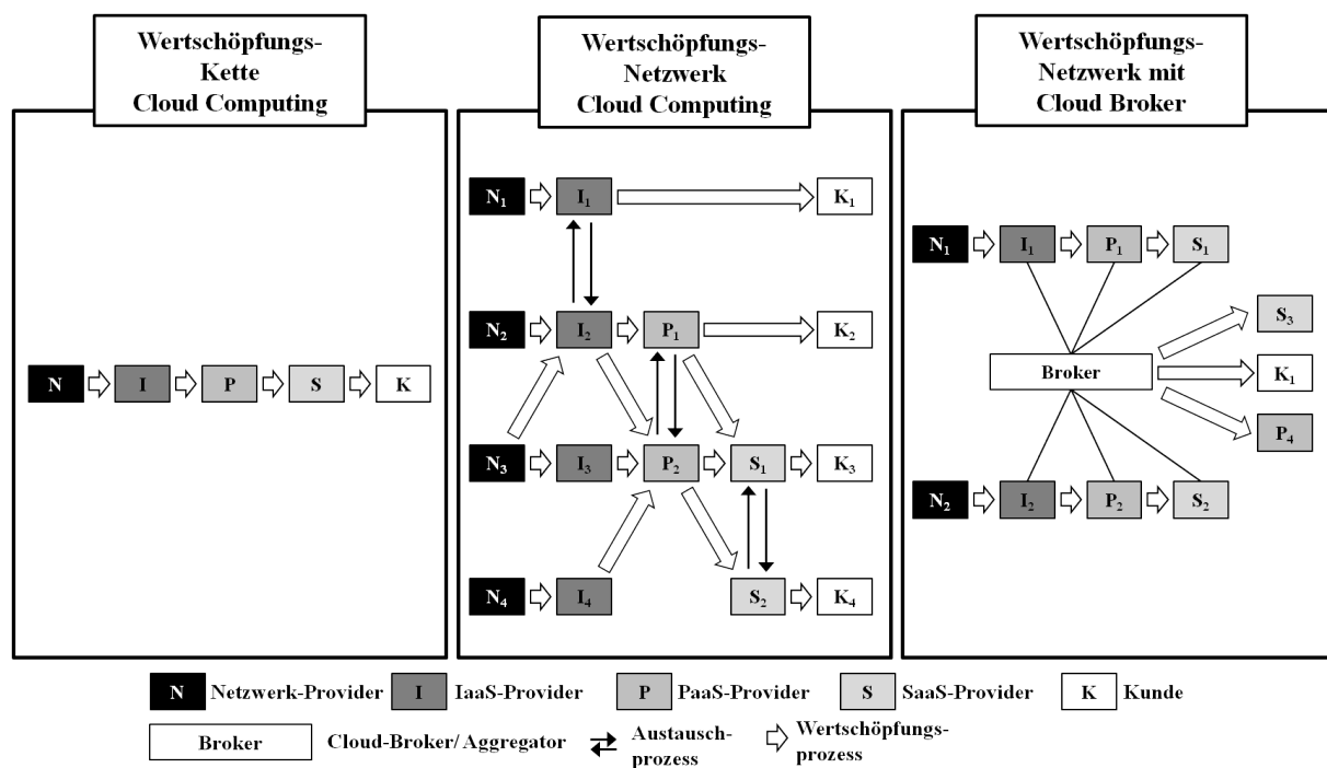
Abbildung 3: Wertschöpfungsnetzwerk Cloud-Computing 17
