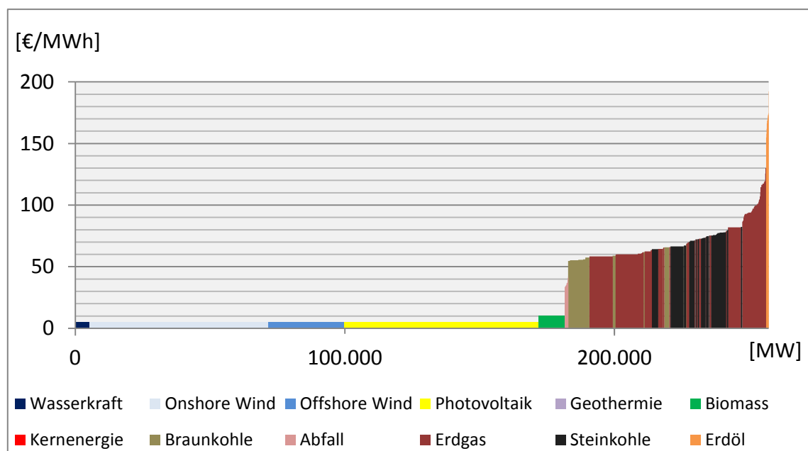
Abbildung 2: Merit Order für Deutschland im Jahr 2032
