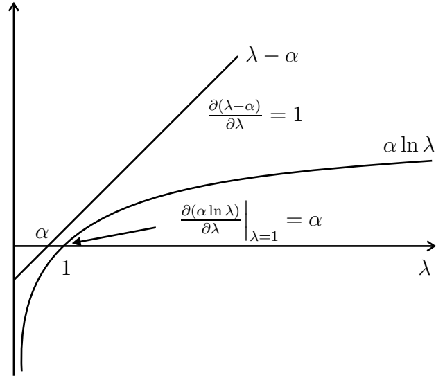
Abbildung 7: \lambda - \alpha > \alpha \ln \lambda für 0 < \alpha < 1 .
