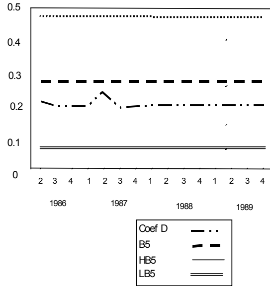
Figura 17 RTCOP (-1)
