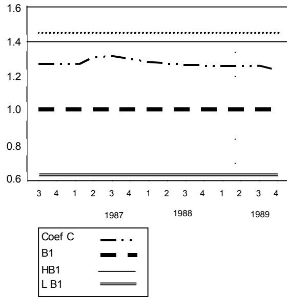
Figura 5 CONSTANTE
