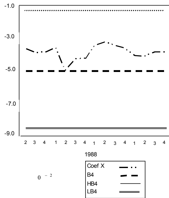
Figura 21 RADESM2
