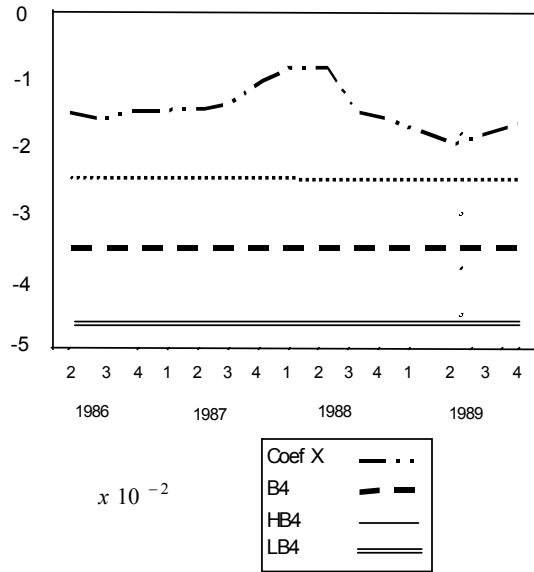
Figura 16 M 1
