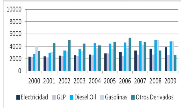
Figura 5: Producción de energía secundaria por energético (en Kbp)
