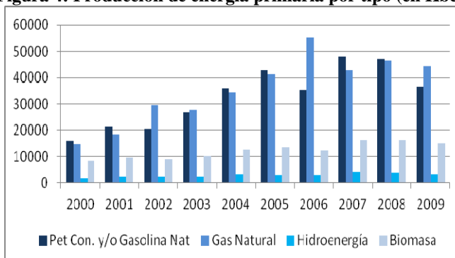
Figura 4: Producción de energía primaria por tipo (en Kbp)
