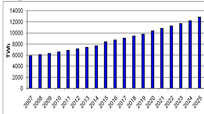
Figura 15. Generación bruta de Electricidad 2007-2025
