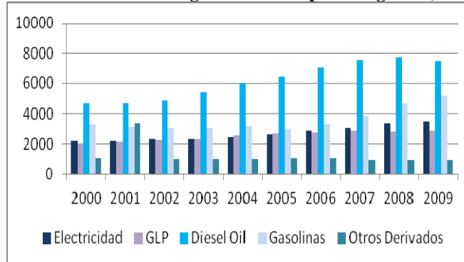
Figura 6: Consumo de energía secundaria por energético (en Kbp)
