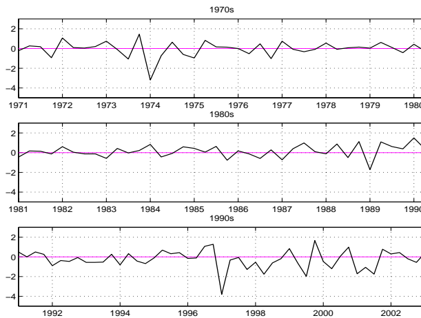
FIG. 6. Output Shocks
