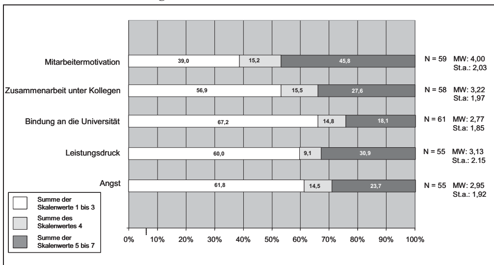
Abb. 4: Häufigkeitsverteilung und Mittelwertanalyse zu den Auswirkungen der Mitarbeiterbeurteilung auf die Mitarbeitenden
