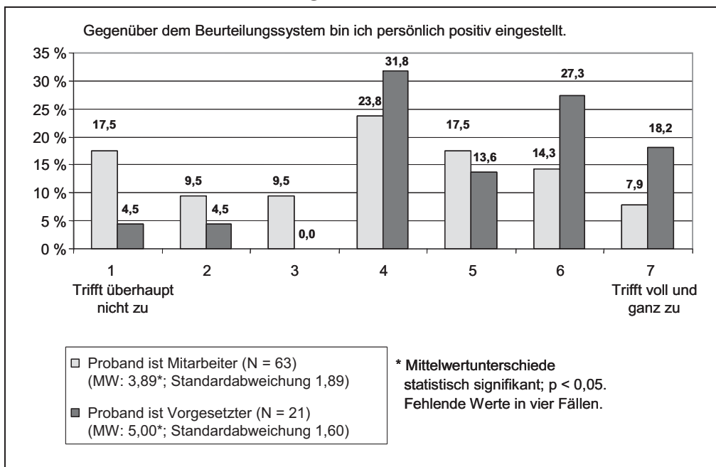
Abb. 3: Mittelwertanalyse zur Überprüfung der Akzeptanz der Mitarbeiterbeurteilung bei Mitarbeitenden und Vorgesetzten
