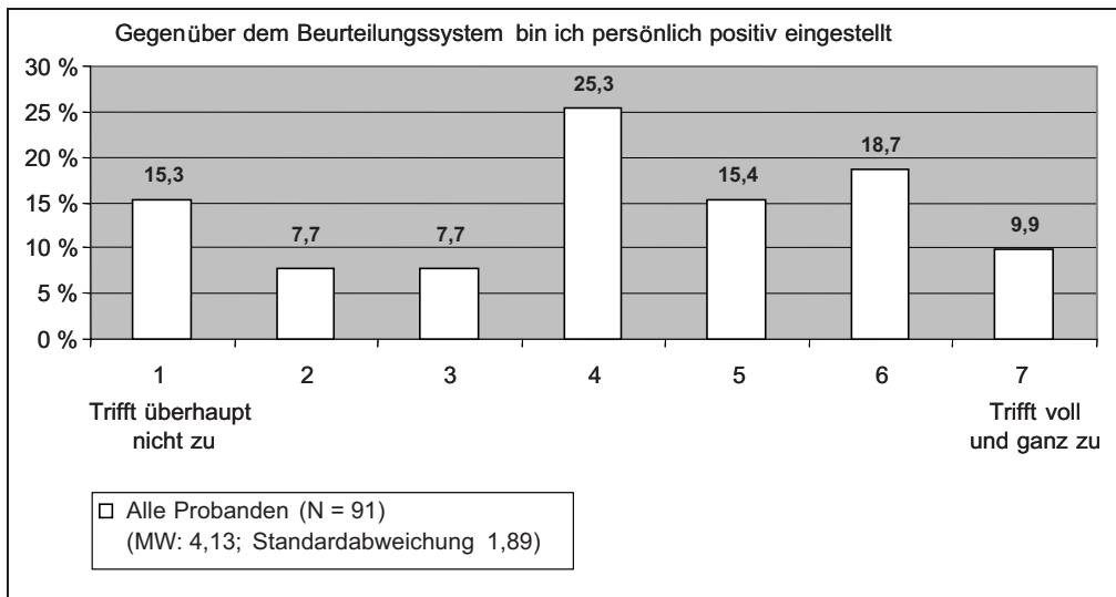
Abb. 2: Mittelwertanalyse zur Überprüfung der Akzeptanz der Mitarbeiterbeurteilung über alle Probanden
