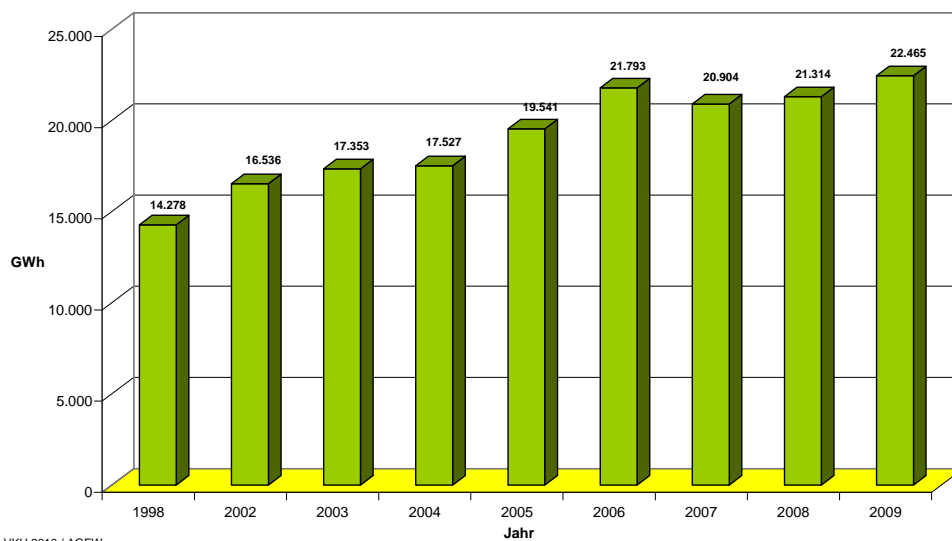
Entwicklung der elektrischen Arbeit der kommunalen KWK-Anlagen 1998-2009
