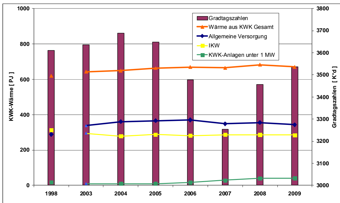
Abbildung 8-1 Gradtagszahlen und KWK-Wärmeerzeugung
