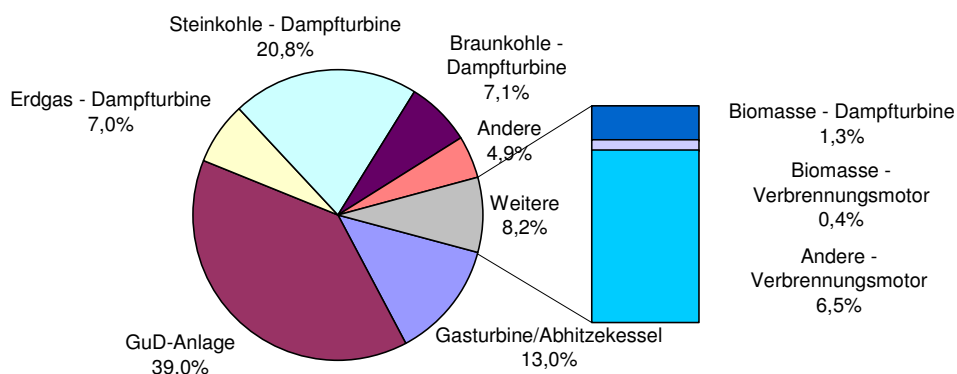
Abbildung 3: KWK-Stromerzeugung der Anlagen der allgemeinen Versorgung nach Maschinenarten und Brennstoffen im Jahr 2008
