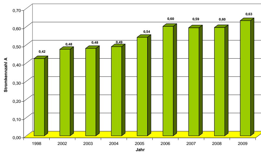
Entwicklung der Stromkennzahl A (elektr. Arbeit KWK / Wärmenetzeinspeisung KWK) für kommunale Anlagen, 1998-2009
