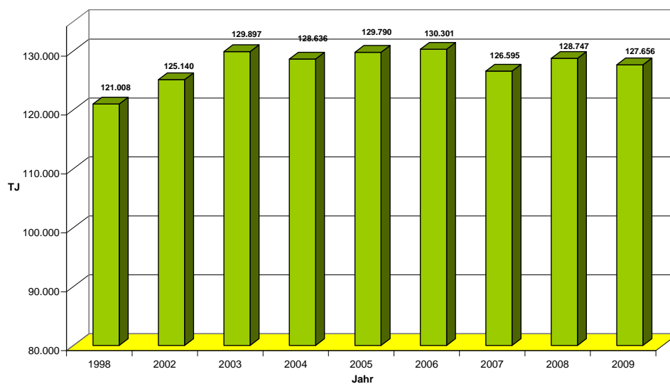
Entwicklung der Wärmenetzeinspeisung aus kommunaler KWK 1998-2009
