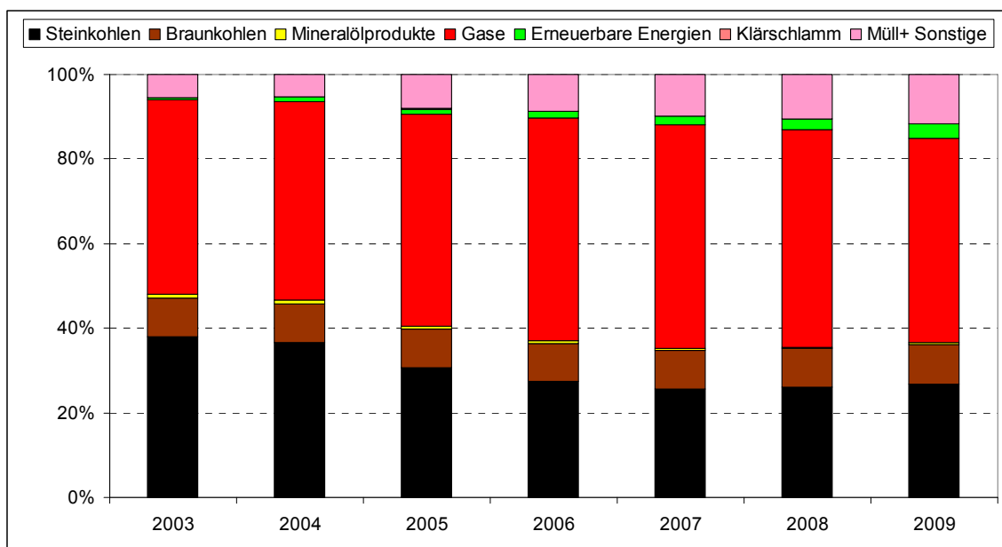
Abbildung A - 1: Brennstoffmix der KWK-Stromerzeugung der allgemeinen Versorgung, 2003-2009
