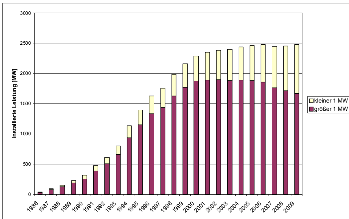
Abbildung 7-1 Installierte Leistung von fossil betriebenen BHKW mit Stilllegung nach 15 Jahren
