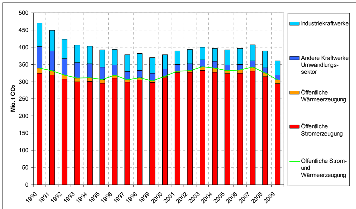
Abbildung 2-1: CO 2 -Emissionen der Stromerzeugung sowie der öffentlichen Strom- und Wärmeerzeugung von 1990 bis 2009
