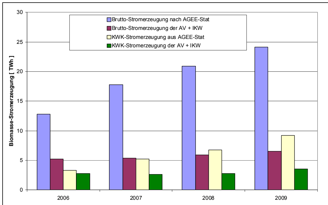
Abbildung 7-2 Entwicklung der Stromerzeugung aus Biomasse nach AGEE-Stat sowie der allgemeinen Versorgung und der industriellen Kraftwirtschaft
