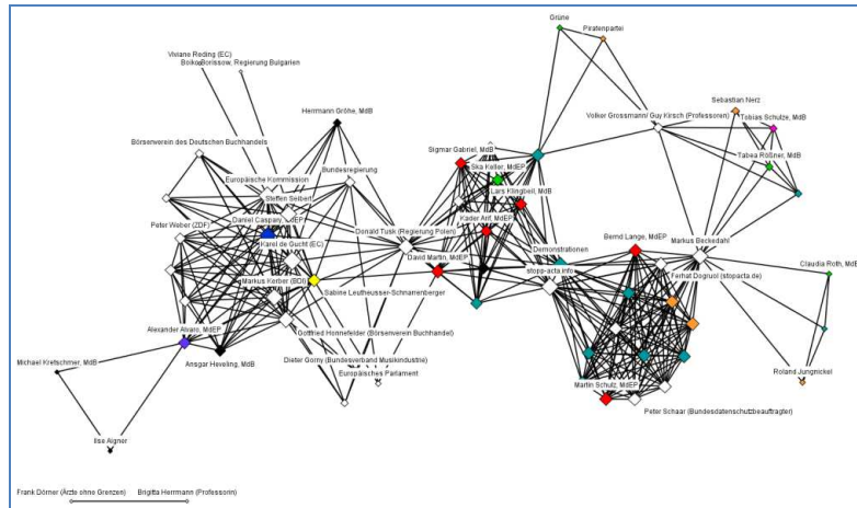
Abbildung 6: Akteur-Kongruenz-Netzwerk März 2012
