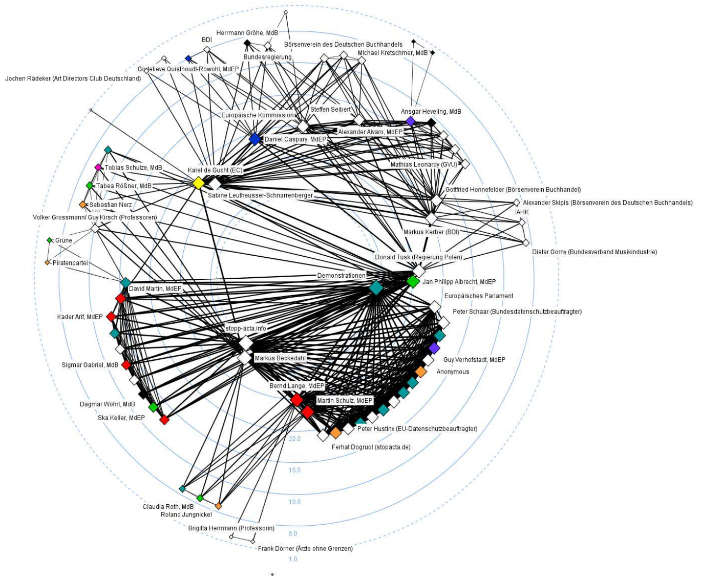
Abbildung 4: Akteur-Kongruenz-Netzwerk
