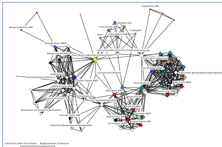
Abbildung 8: Akteur-Kongruenz-Netzwerk Mai 2012
