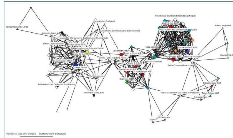
Abbildung 7: Akteur-Kongruenz-Netzwerk April 2012
