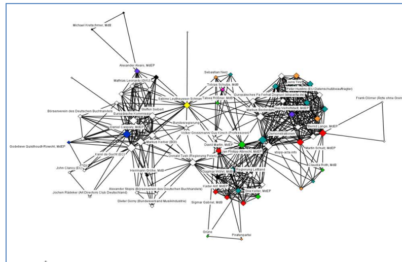
Abbildung 9: Akteur-Kongruenz-Netzwerk Juni/Juli 2012
